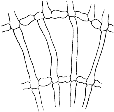
Fig. 3. Querschnitt durch das Aërenchym einer Atemwurzel. Schematisch nach Schenck.
