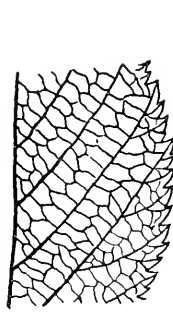
Fig. 3. Schema der craspedodromen Nervatur.
