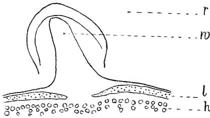
Fig. 2. Schematischer Längsschnitt durch eine Beiwurzel w. r-Rinde, l-Leptom, h-Hadrom des Stengels.
