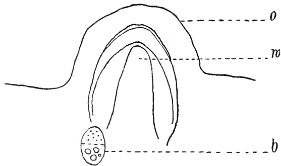
Fig. 9. Schematischer Längsschnitt durch eine Wurzel. o - Epidermis des Stengels, w - Beiwurzel mit Plerom, Periblem, Haube und Wurzeltasche, b - Leitbündel des Stengels.
