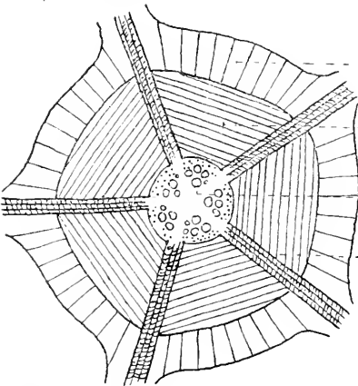
Fig. 6. Schematischer Querschnitt durch einen Knoten. r-äußere Rindenpartie, d-Diaphragma, z-Zentralzylinder, t-Blattbündel.
