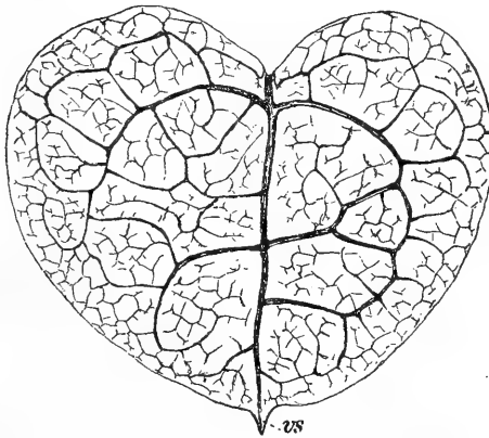
Fig. 26. Nervatur eines Blattes. vs Vorläuferspitze. Vergr. \frac{15}{1} .
