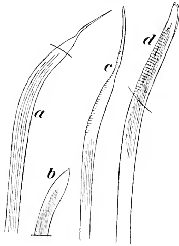
Fig. LIX. Scoloplos hexaphyllum Schm. a = starker, klauenförmiger Haken mit haardünnere Spitze vom oberen Ende des 10. Ventralparapods, im Profil: \frac{2.1.3}{1} . b = distaler Teil eines solchen Hakens, an dem die dünne Endstrecke abgebrochen ist: \frac{2.1.3}{1} . c = kräftige Haarborste mit fast vollständig erhaltener dünner Endstrecke (an der Spitze fehlt ein Stückchen) vom oberen Teil desselben Ventralparapods, im Profil: \frac{2.6.0}{1} . d = schwächerer Haken mit Spitzenscheide vom unteren Teil desselben Ventralparapods, im Profil (der kurze Fortsatz links an der Hakenspitze ist ein Teil der einen, nicht vollständig sichtbaren Scheidenhälfte: \frac{1.0.0}{1} ).
