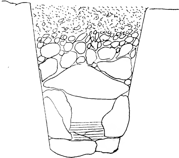
Fig. 100. Steindränage.
