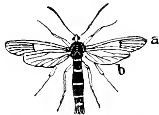
Fig. 2. Mückenähnlicher Glasflügler (Sesiidae), ungefähr zweifach vergrößert. a = Vorder-, b = Hinterflügel.
