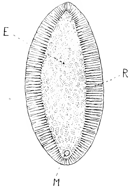
Fig. 18. Ei von Anopheles nigripes nach Eysell (abgeklatscht auf eine fixierte Schicht von Eiweißglyzerin). M = Micropyle, E = Ectochorion, R = Schwimmgürtel. (Aus Archiv f. Schiffs- u. Tropenhyg., Bd. 16.)
