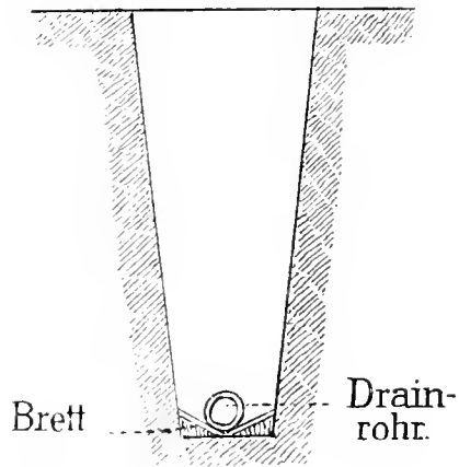
Fig. 95. Röhrendränge mit Holzunterlage (nach Bersch).
