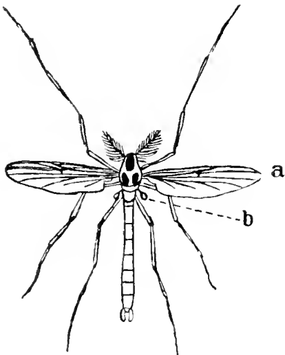
Fig. 4. Zuckmücken ♂ ( Chironomidae ) bei ungefähr zweifacher Vergrößerung. a = Vorderflügel, b = Schwinger.
