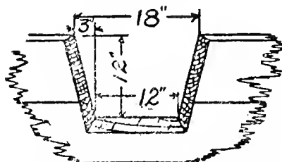
Fig. 5. Trapezoidal or Cipoletti weir.
