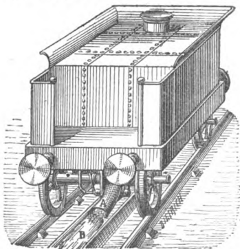
Vorrichtung zum Speisen der Tender mit Wasser ohne Fahrtunterbrechung.
