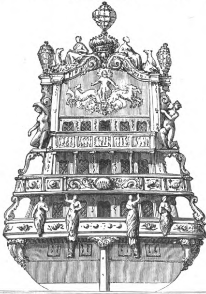
Hinterteil des „Soleil-Royal“ (1690).
