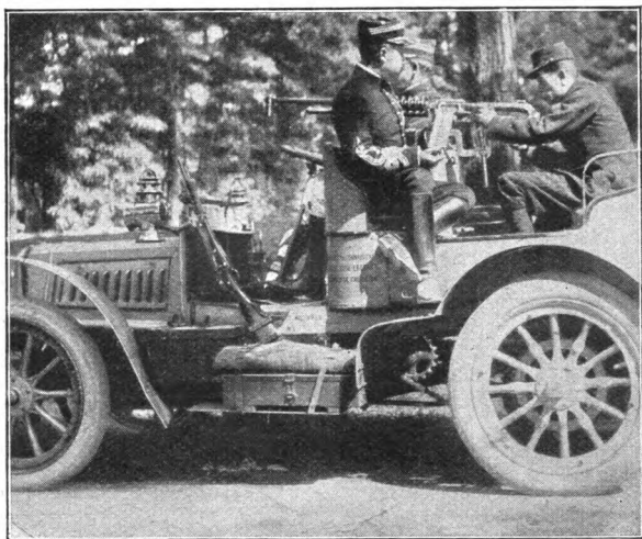
Motorwagen mit einer Hotchkiss-Schnellfeuerkanone. (Französische Armee.)
