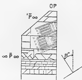
Rhodonitkrystal, sleben \neq \infty \bar{P} \infty , visende spaltbarhed og opbygning. (Fra Westanfors, \frac{24}{9} 1874).
