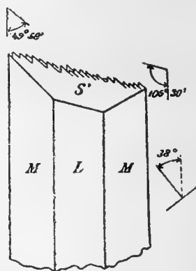
Augitkrystal, type no. 4. (Fra Gammelstilla 1865).
