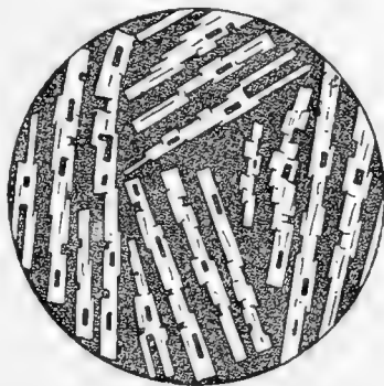
Snit af wollastonit, skaaret \perp paa orthoaxen. (Fra Högfors, 14:de marts 1874 ). (5 o )
