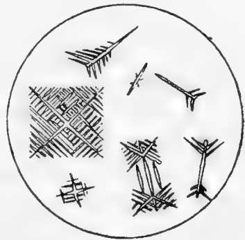
Melilith-mikrolither i en glasrig slag fra Lake superior. ( 3^\circ ).
