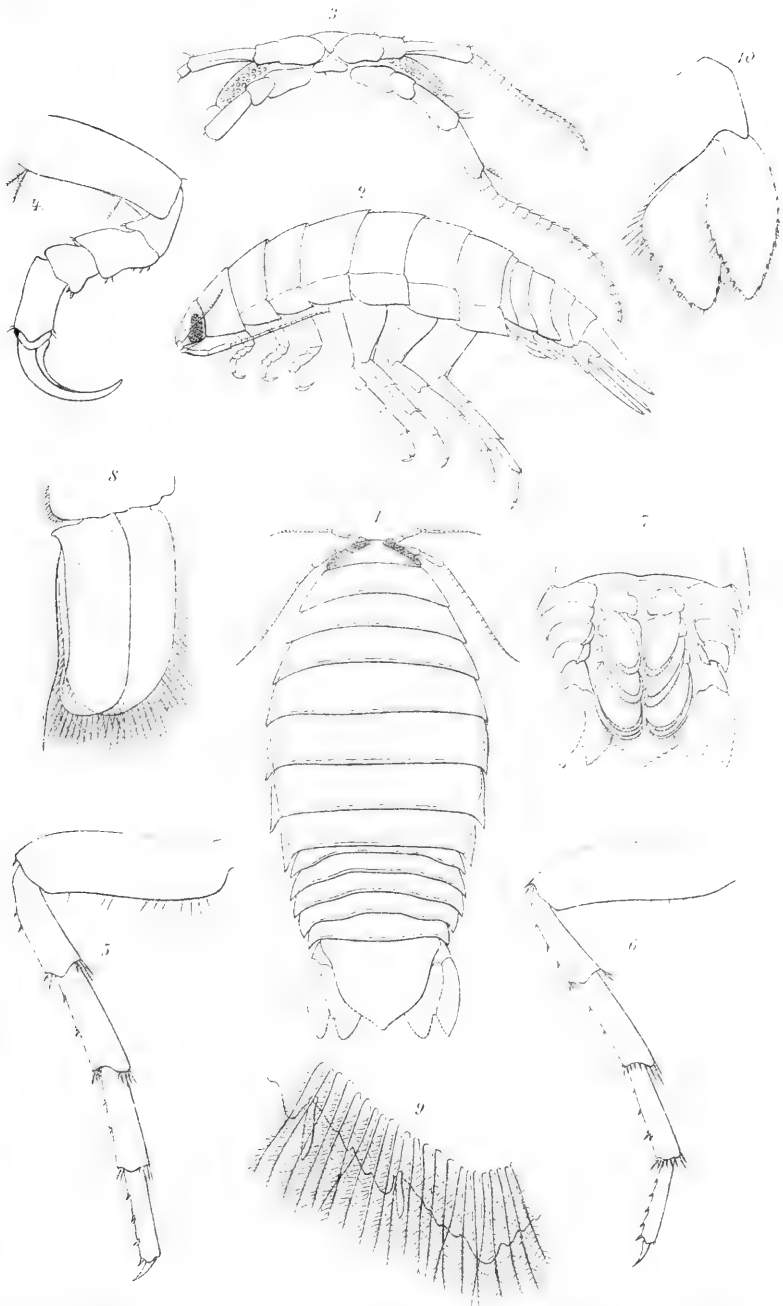
Fig. 1-10. Aega Lovéni n. sp. ♂.
