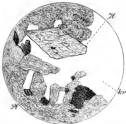
Hornblendekristall H omgifven af kvarts kv, som, förhåller sig som en enhetlig individ. Äfven den starkt sönderdelade plagioklasen visar rätliniga kristallkonturer. Kvartsdioriten fr. Sjögle. Förstor. 40 ggr.
