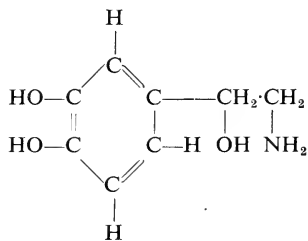
Noradrenaline
