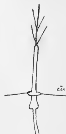
Fig. 9. Schema der Exsudatgrube des Prothorax von P. cucullatus . (Nach Querschnitten kombiniert.)
