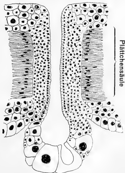
Fig. 3. Drüsig-sensibler Tubulus.
