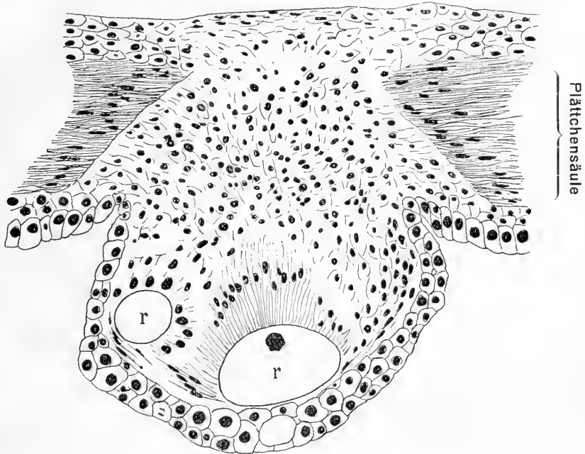
Fig. 4. „Knollenorgane“.
