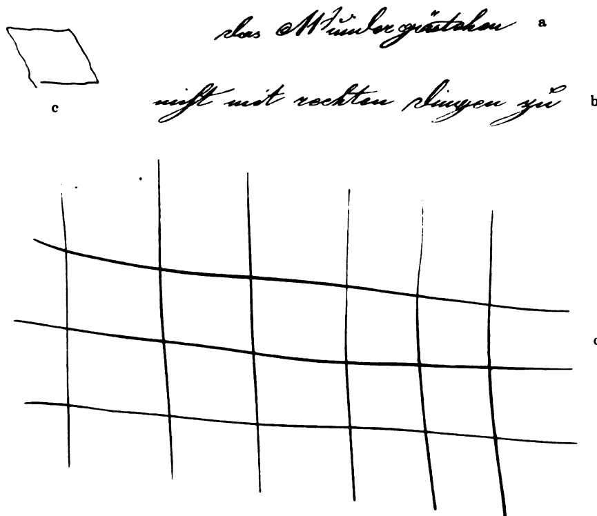
Abb. 1. Schrift und Zeichnung einer Alkoholikerin, deren Tremor gleich auffiel, die ihn aber für Augenblicke unterdrücken konnte. In a ist das Zittern in d , t , h noch zu erkennen. In der Probe b, die aus späteren Zeilen stammt, gar nicht mehr. Beim Zeichnen zittert sie in c noch deutlich, in den großen Zügen von d gelang es ihr, das Zittern ganz zu unterdrücken.
