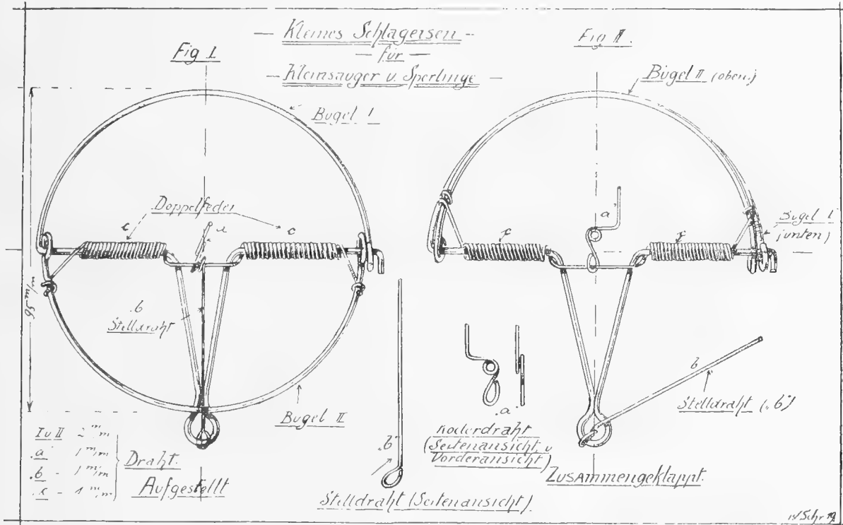
Abb. 2. Kleines Schlagereisen für Kleinsäuger, Sperlinge oder dergl. Skizzen von W. Schreitmüller-Frankfurt a. M.
