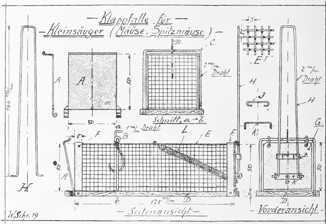
Abb. 1. Klappfalle für Kleinsäuger, wie: Mäuse aller Art, Spitzmäuse zc. Skizze von W. Schreitmüller-Frankfurt a. M.
