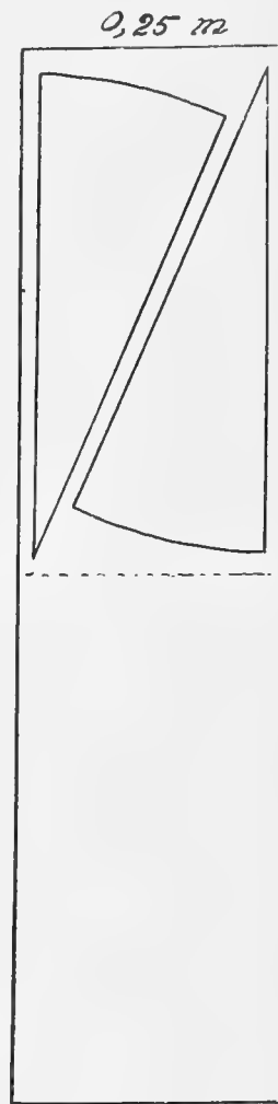
Abb. 5–7. Zur Herstellung eines Schnittmusters für den Gazebeutel.
