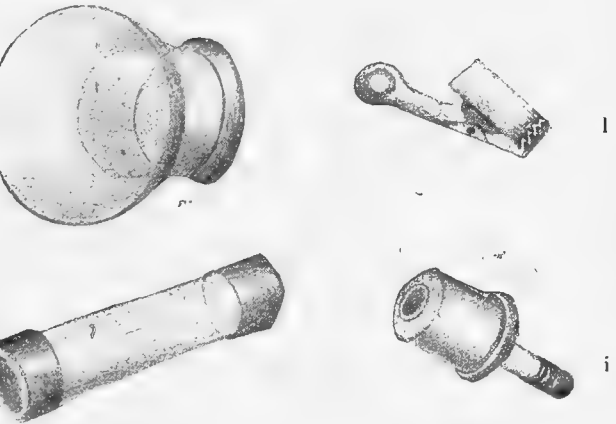
Abb. 4. Einzelne Teile des Planktonnetzes. c. Durchschlag, f. Glasansatz mit 2 Hartgummiringen, i. durchbohrter Pfropfen mit durchführende Metall- röhre, l. Klammer.
