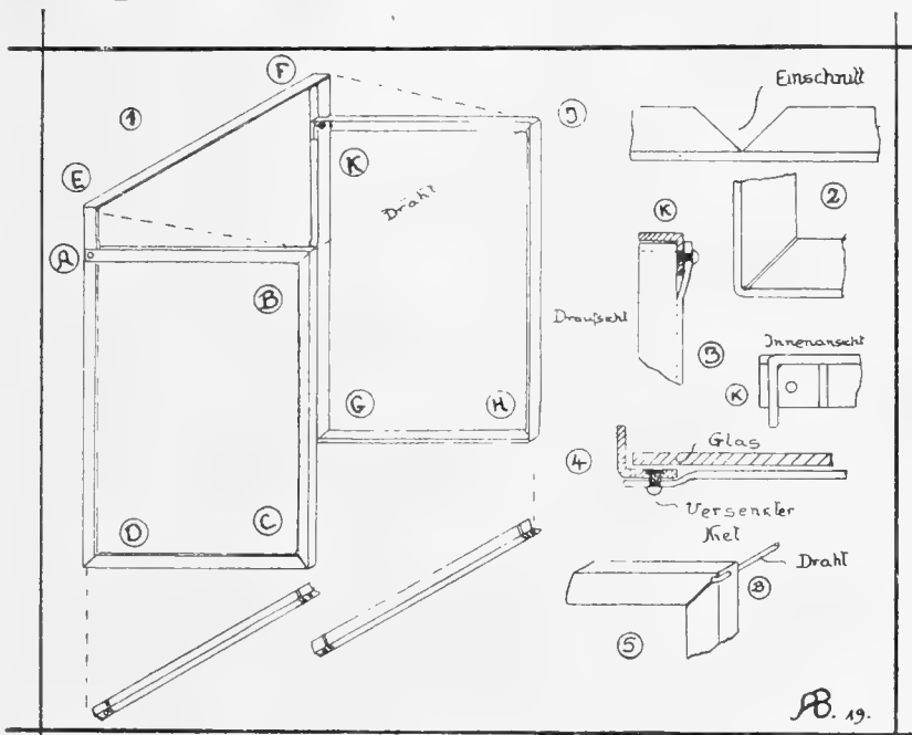
Abb. 2. 1. Einzelteile des Hängeaquariums 1 ; 2. Biegung des Winkeleisens; 3. Vernietung bei A und K; 4. Befestigung der Seile CH und DG an den Pfosten; 5. Befestigung des Drahtes bei B und J.
