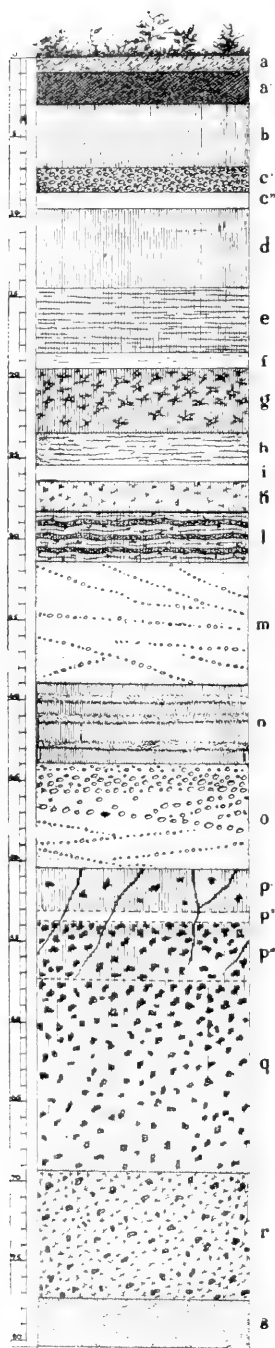
Fig. 1. — Pleistoceno de Córdoba
