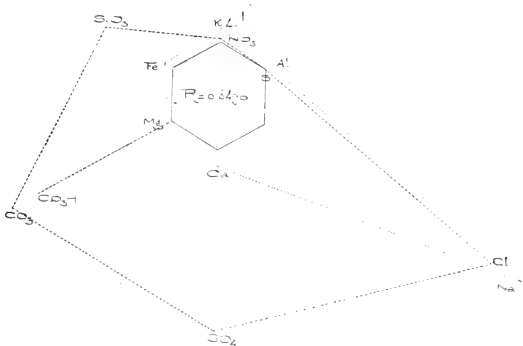
Arroyo Confluencia (termas de Inti) t = 38^{\circ}C
