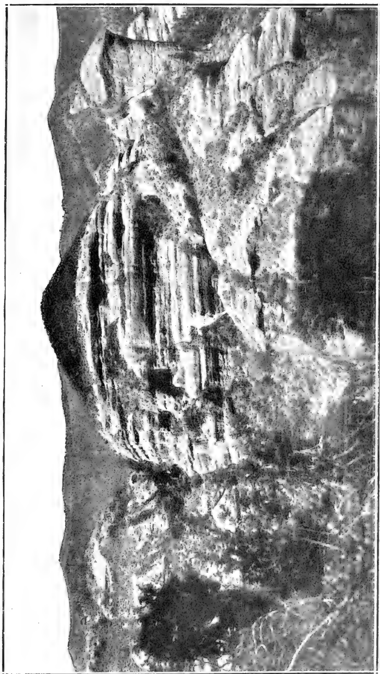
Fig. 3. — Los terranos de la Quebrada de Lama. Estratos de Paganzo, areniscas trinitarias
