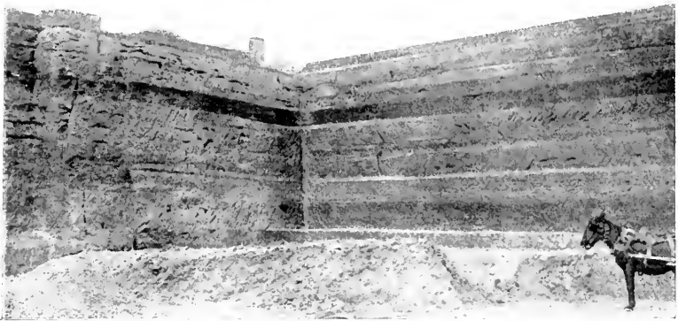
FIG. 1. a —Estratificación horizontal en las arcillas. Desmante junto al puente de Zulema.
