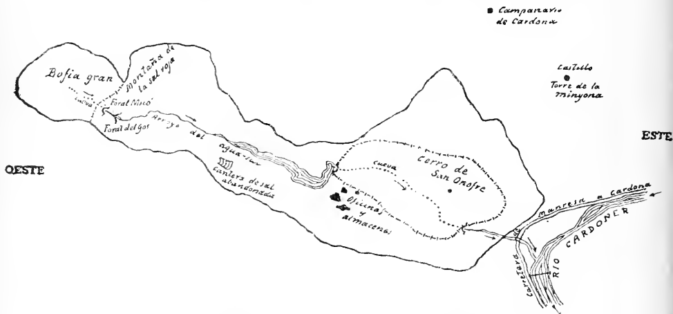
Fig. 1.ª.—Perímetro de la sal descubierta en las salinas de Cardona.
