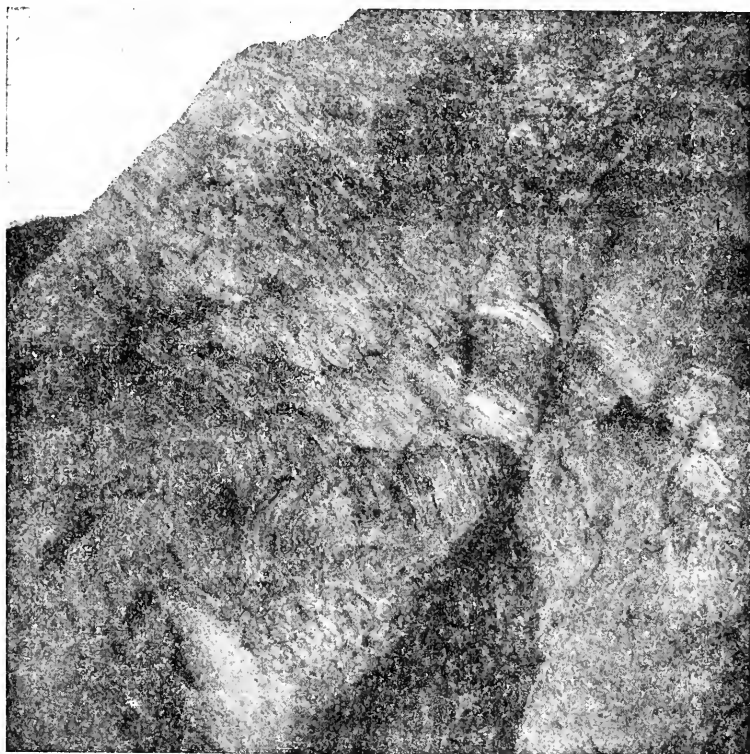
Fig. 4.ª—Pliegues curvos en la sal por el camino de la Bofia gran.
