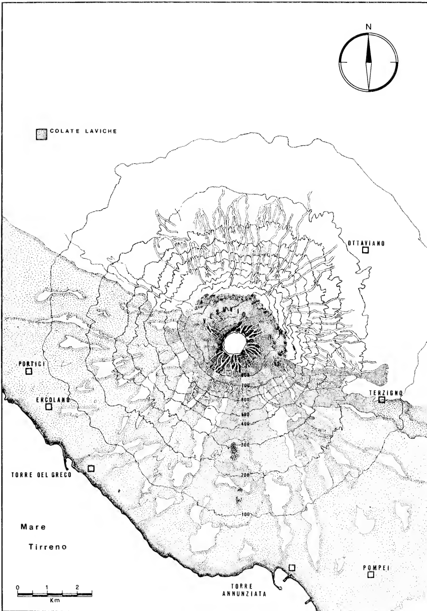
FIG. 2. - Altimetria del complesso Somma-Vesuvio e colate laviche delle più recenti eruzioni.
