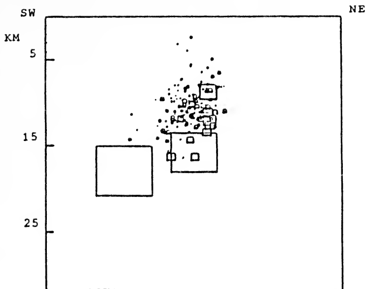
FIG. 3. — Distribuzioni ipocentrali con orientazioni: SN, SE-NW, SW-NE. Le dimensioni dei quadrati sono proporzionali alle magnitudo e sono relativi agli eventi sismici di classi A e B (secondo HYP071).
