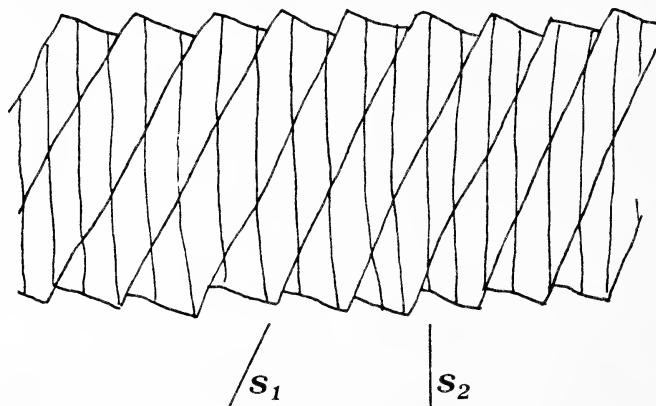
FIG. 4. — Doppio sistema di clivaggio in uno strato. Il sistema S_2 è paleamente posteriore a quello S_1 .
