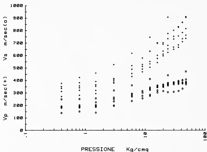
FIG. 6. — Andamento delle variazioni di V_p (+) e V_s (0) in funzione della pressione verticale per i campioni di pozzolana allo stato naturale.
