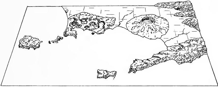
FIG. 1. - Posizione del sistema Somma-Vesuvio nella conca napoletana.
