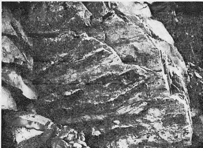
FIG. 5. — Superficie attuale di uno strato su cui si distinguono vene di calcite fibrosa disposte in bande parallele alle tracce delle superfici di clivaggio. L'allungamento dei cristalli e le sliccoliti presenti sul calcare esposto sono parallele alla direzione di scivolamento degli strati.
