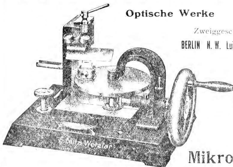
Rotationsmikrotom
