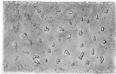
Fig. 2. Aphanizomenon flos aquae . Schwebekörper, nach längerem Liegen der Zellen in 10% Kalisalpetere-lösung durch Druck isolirt. Vergrösserung etwa 700.
