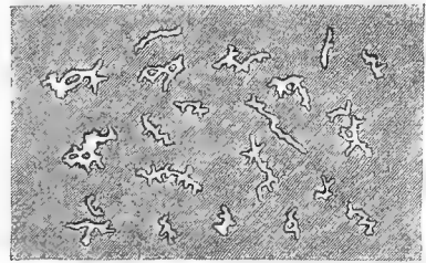
Fig. 4. Aphanizomenon flos aquae Ralfs. Grössere Massen von Schwebekörpern, entstanden durch spontane Verschmelzung von kleineren. Vergrösserung etwa 700.
