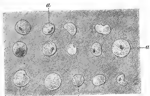
Fig. 3. Aphanizomenon flos aquae Ralfs. Vacuolen mit Schwebekörpern und ausserordentlich kleinen in Brown'scher Molecularbewegung begriffenen Kügelchen. In 4% Kalisalpeterlösung isolirt. Vergrösserung etwa 1200.
