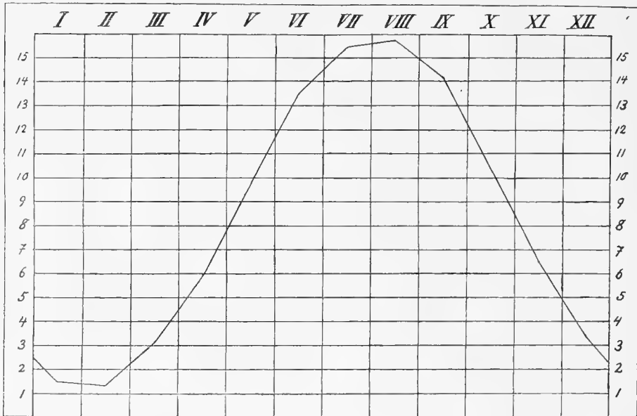
Fig. 1. Temperaturmittel (monatlicher Durchschnitt) von 15 Jahren (1893—1907) für Helgoland.
