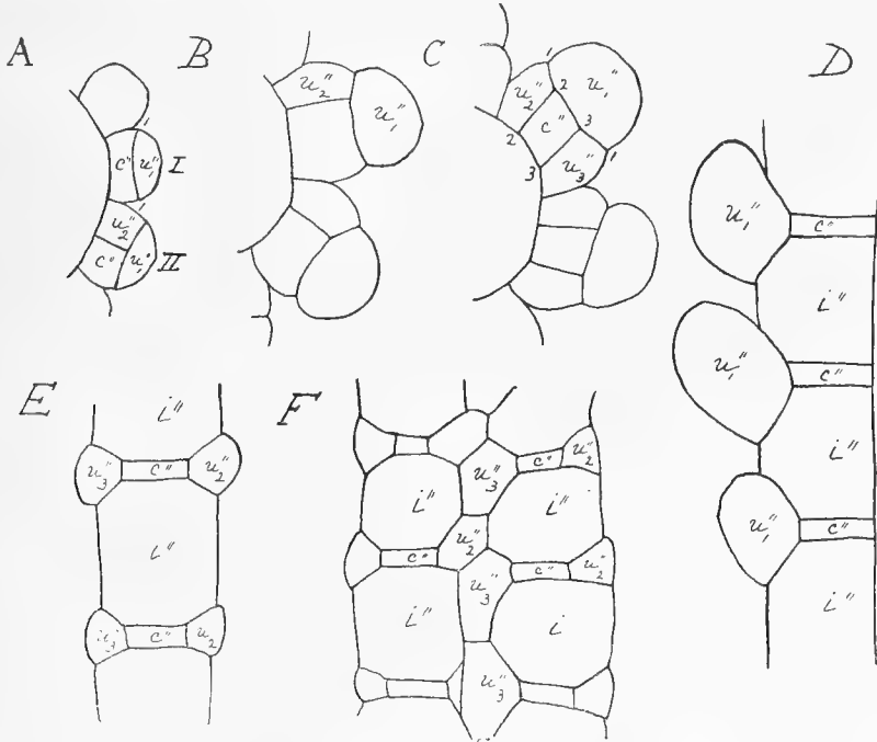
Fig. 7. Chara contraria . A—C Querschnitte durch Rindenrippen in verschiedenen Stadien der Entwicklung. D Längsschnitt durch einen Rindenrippenschlauch. E F Tangentialschnitte durch Rindenrippenschläuche. Ausbildung der Zwischenreihen. Vergr. 240:1.
