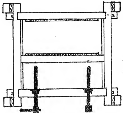
Fig. 2.—Plan.
