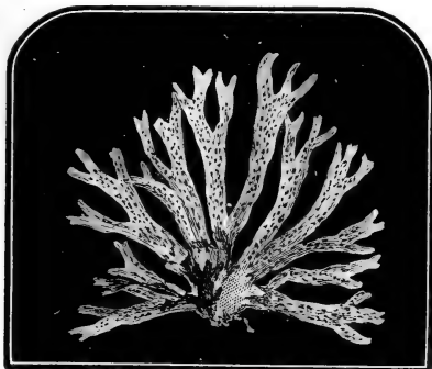
FIG. 123. Nitophyllum punctatum , var. Ocellatum .
