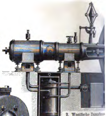
2. Woolfsche Dampfmaschine
