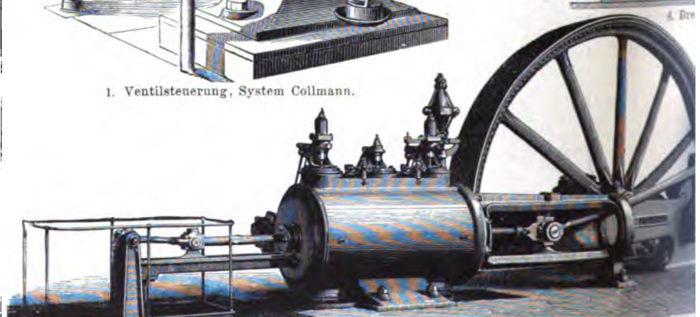
7. Ventil-Dampfmaschine von Sulzer.
