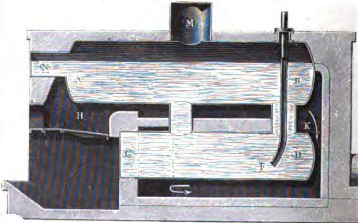
1. Gewöhnlicher Dampfkessel mit Vorwärmer.
