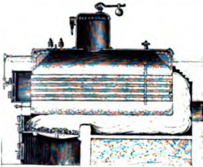
19. Kessel mit Feuerröhren, Längsschnitt.
