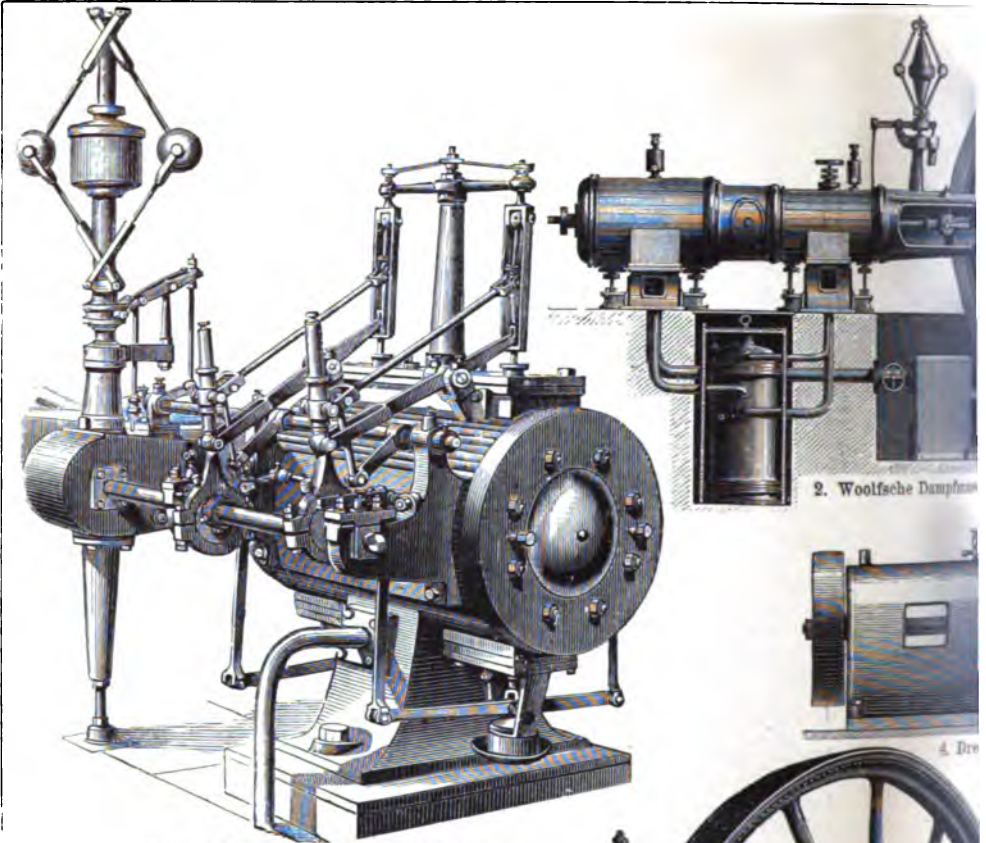
1. Ventilsteuerung, System Collmann.
