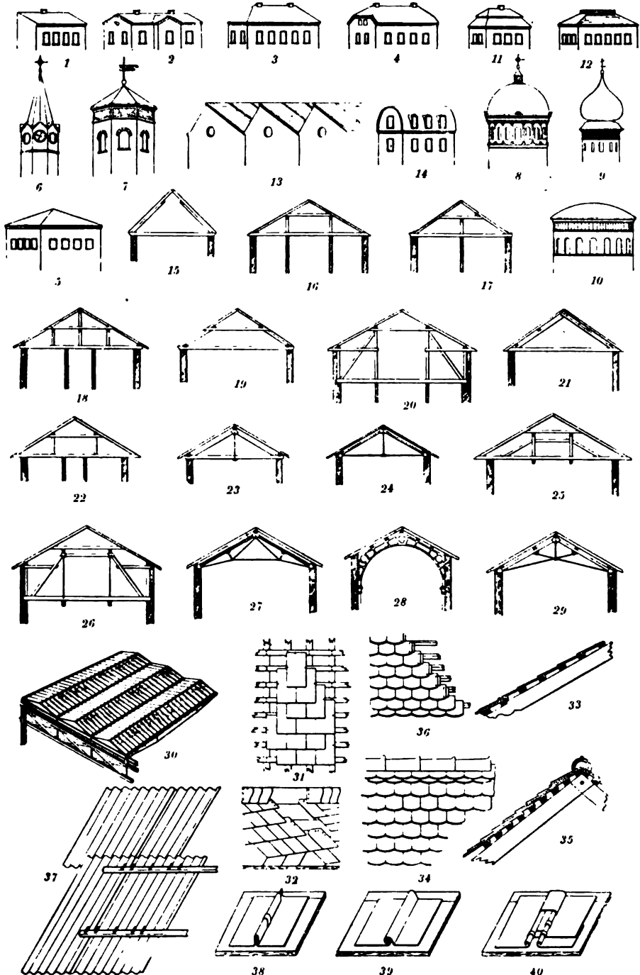
1. Fultdach. 2. Satteldach (mit Giebeln). 3. Walmdach. 4. Halber Walm. 5. Zeltdach (quadratisch). 6. Helm. 7. Zeltdach (polygonal). 8. Kuppeldach. 9. 10. Dachhaube. 11. Mansarde. 12. Terrassen- oder Plattform- dach. 13. Sheddach. 14. Bohlendach. 15. Dach mit Windrispe. 16. Doppeltstehender Dachstuhl. 17. Ein- fachstehender Dachstuhl. 18. Dreifachstehender Dachstuhl. 19. Liegender Dachstuhl. 20. Pfettendach mit stehendem Dachstuhl und versenktem Gebälke. 21. Reines Pfettendach. 22. Pfettendach mit stehendem Dachstuhl. 23. 24. Pfettendach mit einfachem Hängewerk in Holz- und Eisenkonstruktion. 25. Kehl- balkendach mit doppeltem Hänge- und Sprengwerk. 26. Kehl- balkendach mit doppeltem Hänge- und Sprengwerk, mit Eisenkonstruktion und versenktem Gebälke. 27. Dach in Eisenkonstruktion (sog. Polonceau). 28. Dach- konstruktion in Gufeisen. 29. Pfettendach mit Eisenkonstruktion (deutsches System). 30. Dach in Eisen- und Glas. 31. Schieferdach (englisch, doppelt). 32. Schieferdach (deutsch). 33. 34. Ziegeldach, einfach. 35. 36. Ziegeldach, doppelt. 37. Wellblechdachung. 38. 39. 40. Zinkbedachung mit Falzen, Rollen und Deckblechen.
