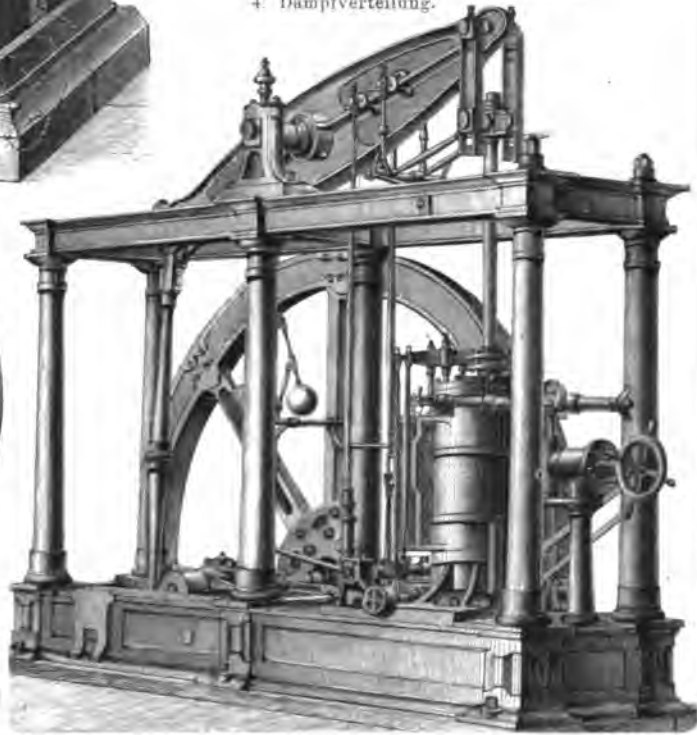
8. Maschine mit Balancier nach Watt.
