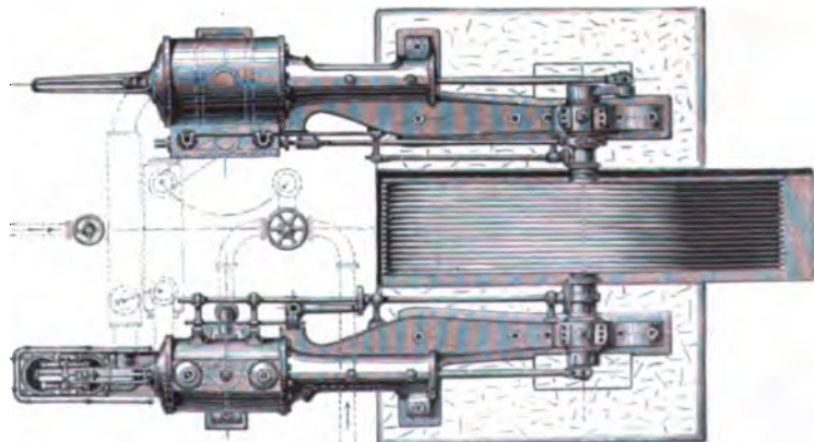
10. Compound-Dampfmaschine von Collmann.
