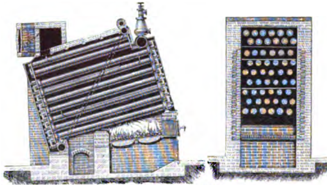
14. 15. Rootscher Kessel.
