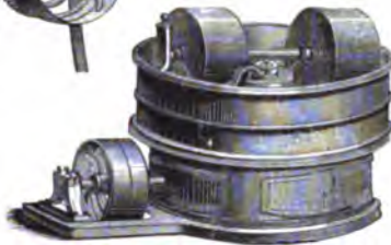
5. Melangeur mit rotierendem Bodenstein.
