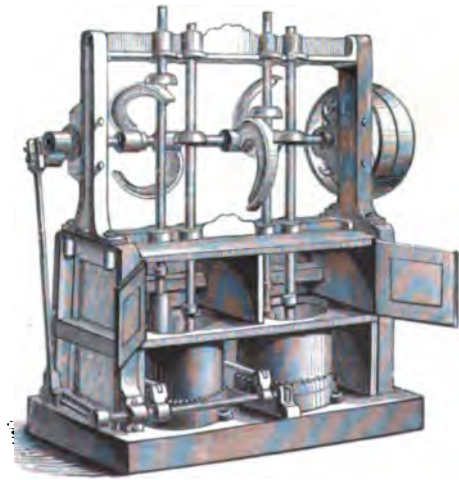
8. Stampfwerk.
