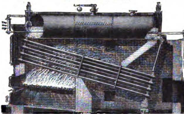
11. Dampfkessel von Babcock & Wilcox.
