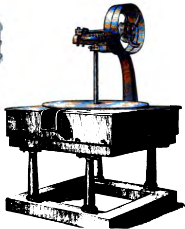
7. Dampf-Röstmaschine.
