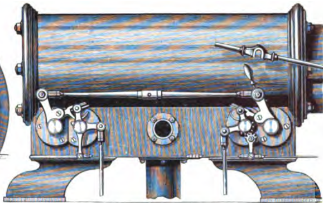
3/ Corliss-Steuerung, System Wheelock.
