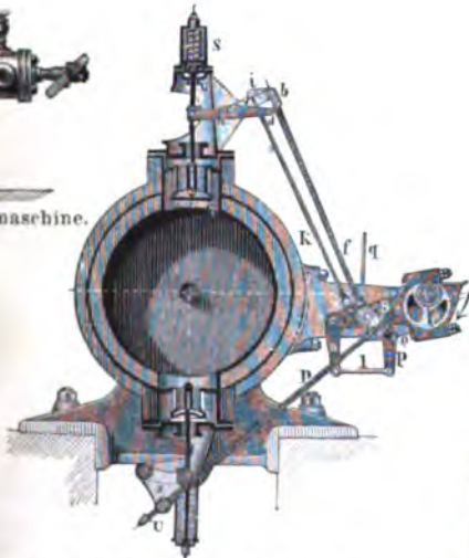
5. Ventilsteuerung, System Sulzer.
