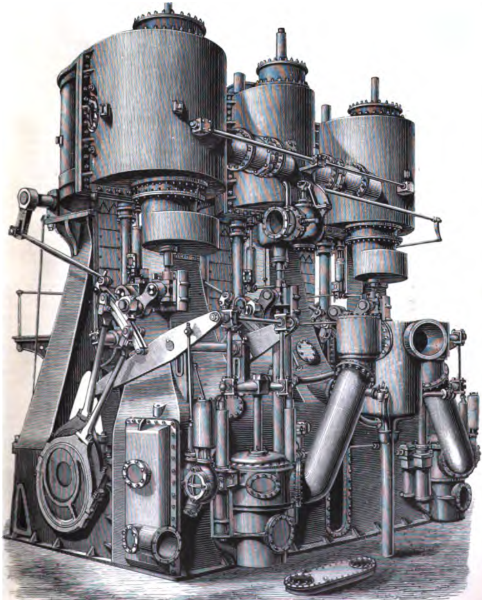
1. Seitenansicht einer dreieylindrigen Compound-Schiffsmaschine.
