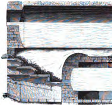
6. Etagenrost von Langen.
