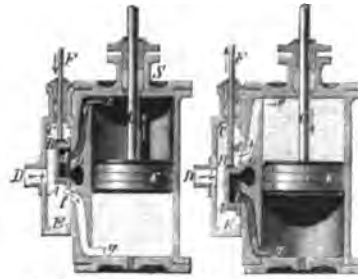
4. Dampfverteilung.
