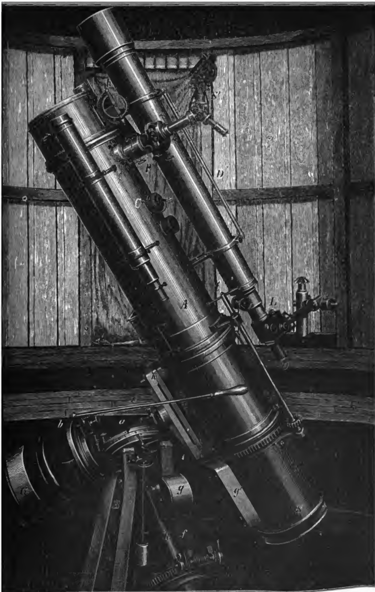
Fig. 17. E. von Gothard's Spiegeltelescop von J. Browning.
