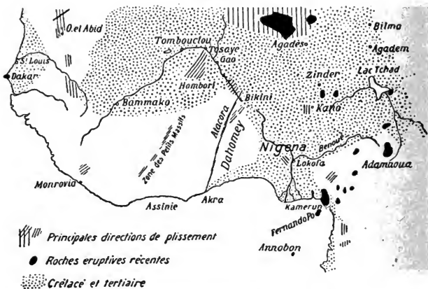
Streichrichtungen in Afrika, nach Lemoine.
