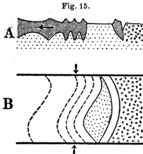
Schema der Entstehung von Inselgirlanden. A Querschnitt; B Aufsicht. (Der stark ausgekühlte Teil des Sima ist durch Strichelung bezeichnet.)
