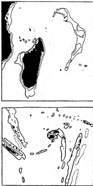
Oben: Madagaskar und Seychellen-Bank. Unten: Die Fidschi-Inseln. (Tiefenlinien 200 und 2000 m; Tiefseerinnen punktiert.)
