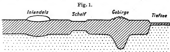
Schnitt durch die Lithosphäre nach der Isostasielehre.
