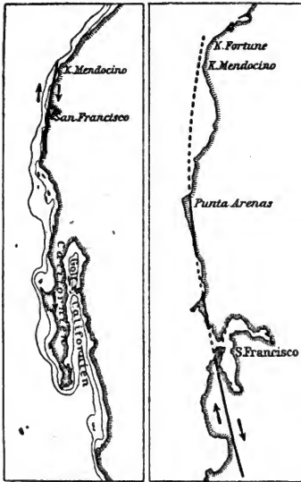
Kalifornien und die Erdbebenverwerfung von San Franzisko.
