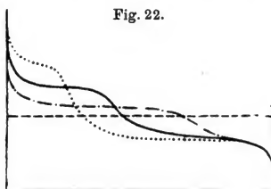
Fig. 22. Ehemalige und künftige hypsometrische Kurve der Erdoberfläche. .... für die Zukunft, — für die Gegenwart, - - - für die Vorzeit, — — im Urzustand (zugleich mittleres Krustenniveau).
