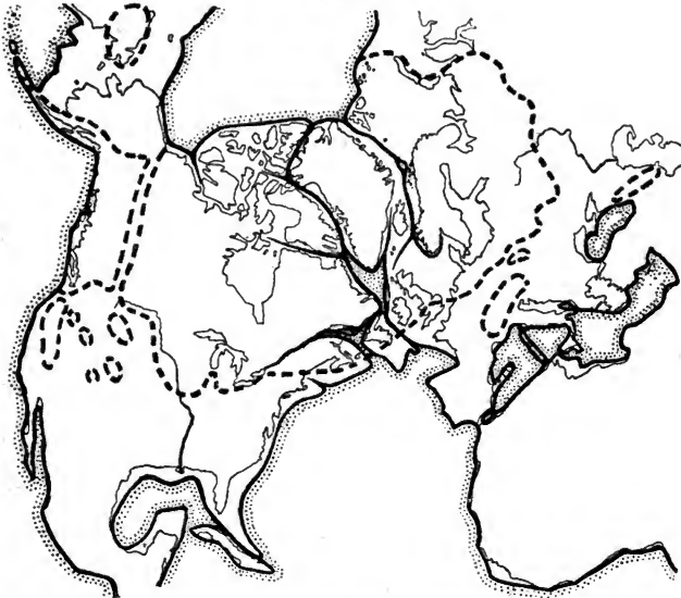
Rekonstruktion der Kontinentalschollen für die große Eiszeit.
