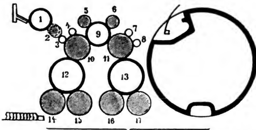
Fig. 109. (Querschnitt eines sogenannten doppelten Farberkes an Buchdruckmaschinen für monochromen Druck. 1, 3, 4, 7, 8, 9, 12 und 13 sind Stahlwalzen; 2, 5, 6, 10, 11, 14, 15, 16 und 17 sind Massewalzen.)
