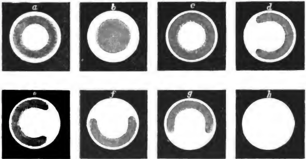
Fig. 30. Centrirung der Lichtquelle.
