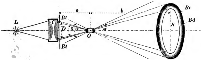
Fig. 31. L = Lichtquelle. C = Condensator, D = Platte (Diapositiv), BI = Plattenträger als Blendenebene ausgebildet, O = Objectiv, o = Objektweite, b = Bildweite, \alpha = thatsächlicher Bildwinkel des Objectives, \delta = erforderlicher Bildwinkel, um ein Bildfeld ohne Farbensaum zu erhalten, S = Schirm, Br = Bildkreis = Bild des Randes der Condensatorfassung, Bd = Bildkreis = Bild des Randes der Blendenebene BI .
