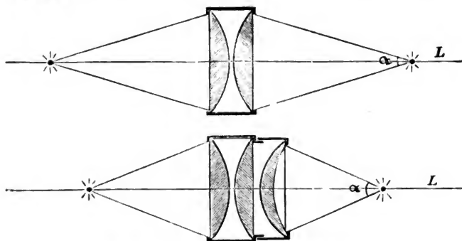
Fig. 29. L = Lichtquelle, \alpha = Oeffnungswinkel.
