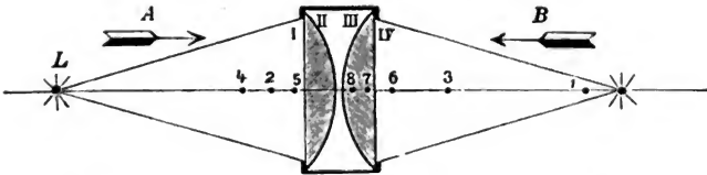
Fig. 32. L = Lichtquelle; I II III IV = Flächen der Condensatorlinsen; 1 bis 8 = Lage der Spiegelbilder.
