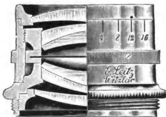
Fig. 62. Anastigmat von E. Leitz.
