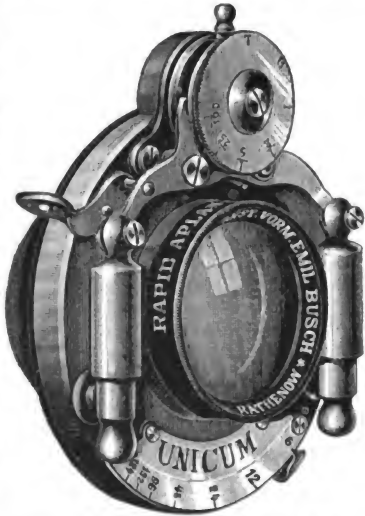
Fig. 19. Rapidaplanat Nr. 2, f/8 , mit Bausch & Lomb's Momentverschluss. Natürl. Grösse.
