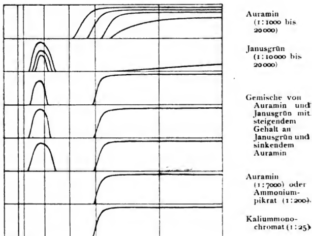
Fig. 73. Absorptionsspectra gefärbter Flüssigkeiten in verschiedenen Concentrationen.
