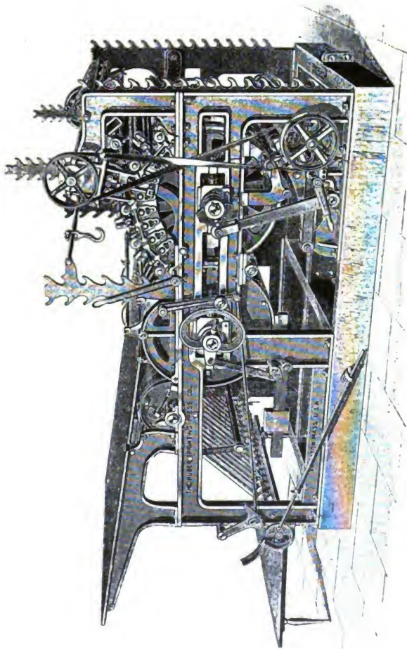
Fig. 84. Amerikanische Presse für Aluminiumdruck.
