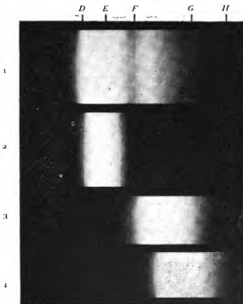
Fig. 71. Spectrumphotographie auf einer Erythrosinplatte (Gaslicht, kleiner Glasspectrograph). 1. Freier Apparat. 2. Vorschaltung einer Lösung von Kalumbichromat und Säuregrün. 3. Lösung von Kupferoxyd-Ammoniak. 4. Lösung von Methylviolett.
