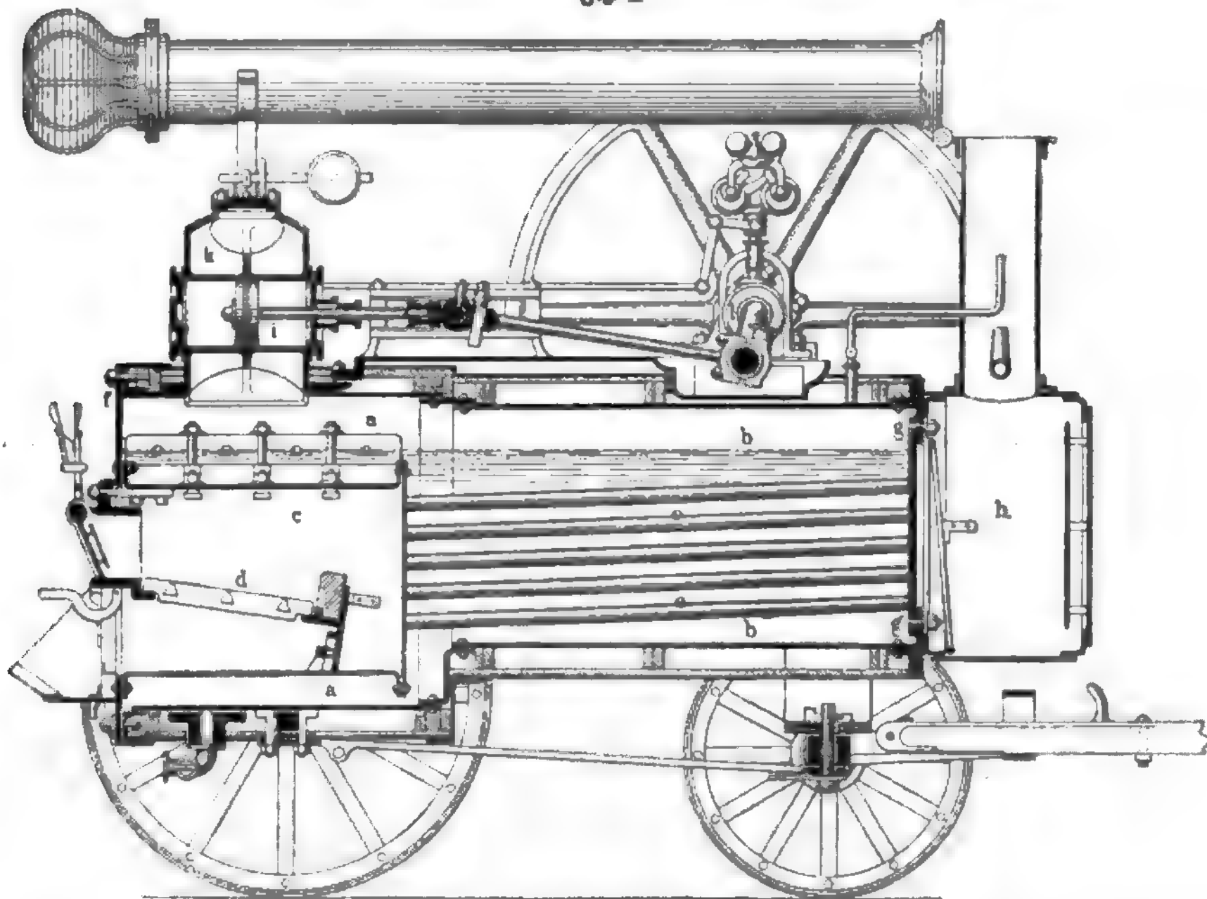
Locomobile von Wolf.
