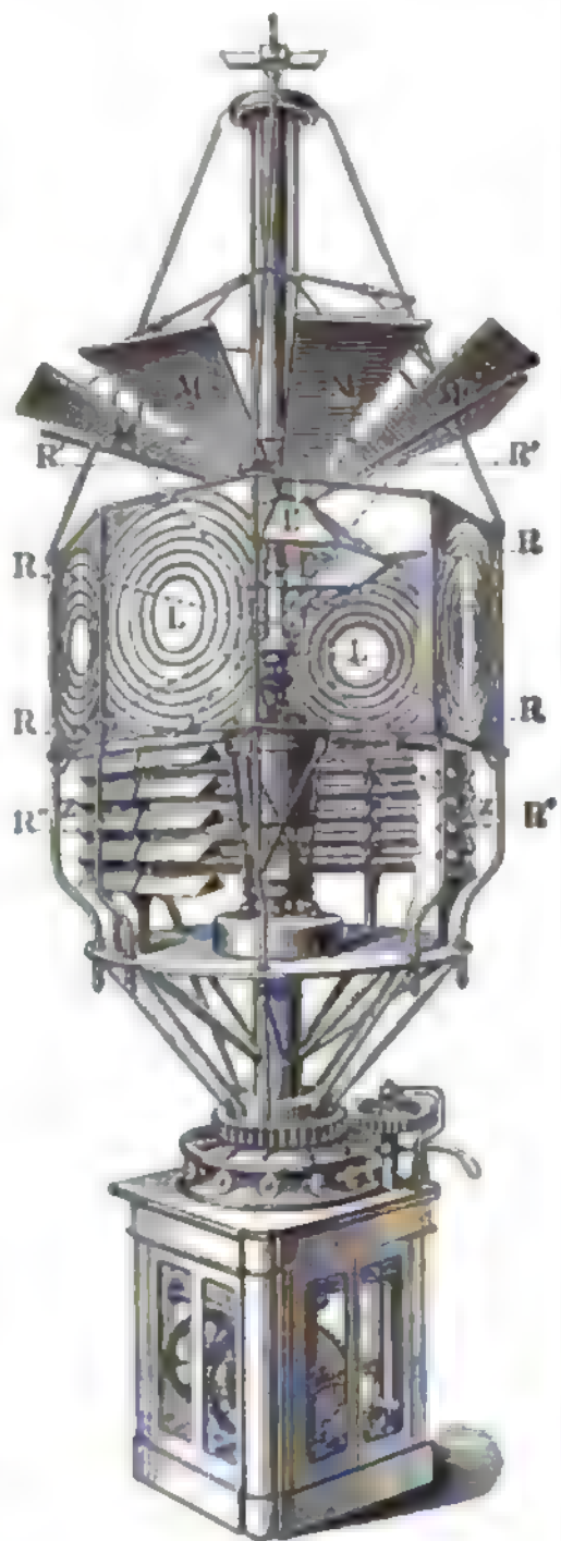
Fig. 4. Leuchtturm mit Drehfeuer.
