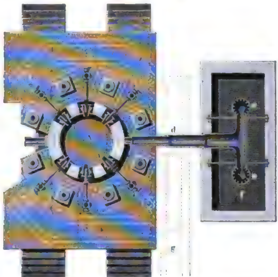
Fig. 2. Mansfeldscher Ofen mit kontinuierlichem Schlackenabfluß. Querschnitt.
