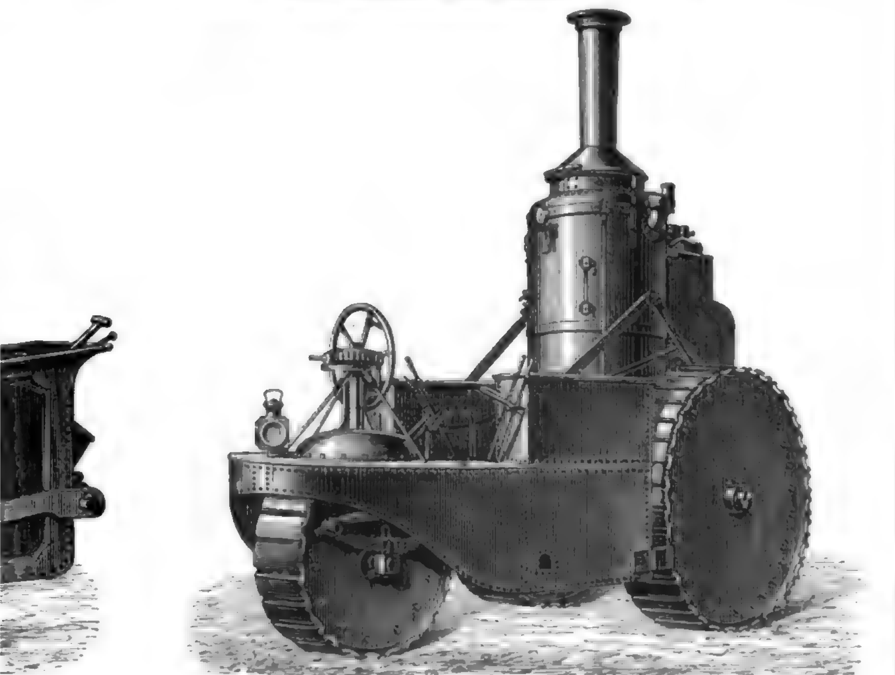
Fig. 4. Straßenlokomotive von Thomson.
