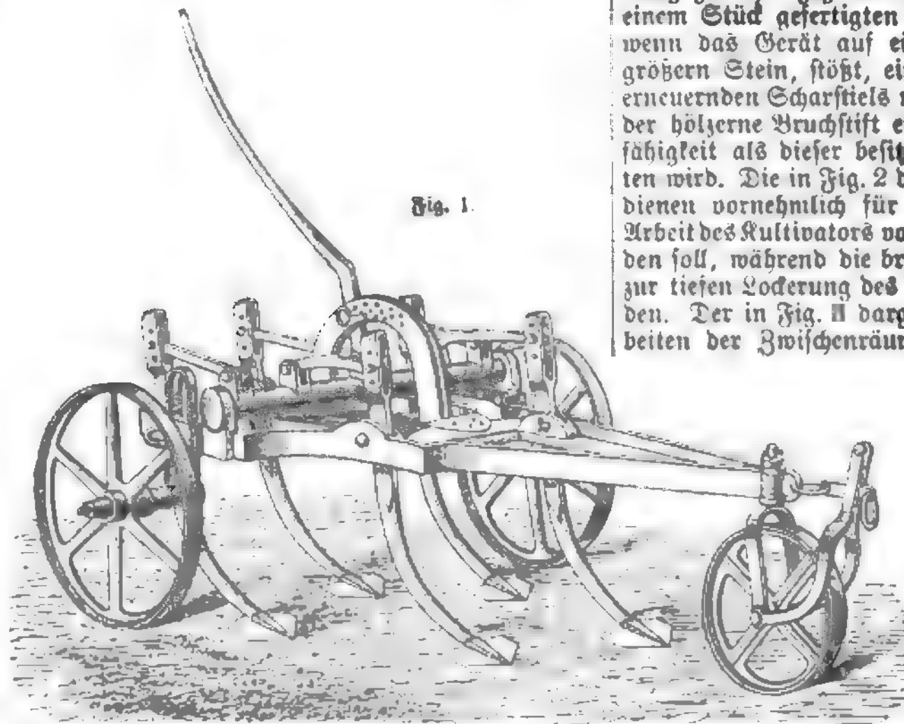
Kultivator von Coleman.
