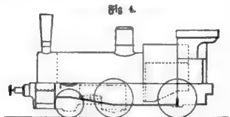
Lokomotive für gemischte Züge.
