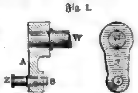
Fig. 1. Stirnkurbel.
