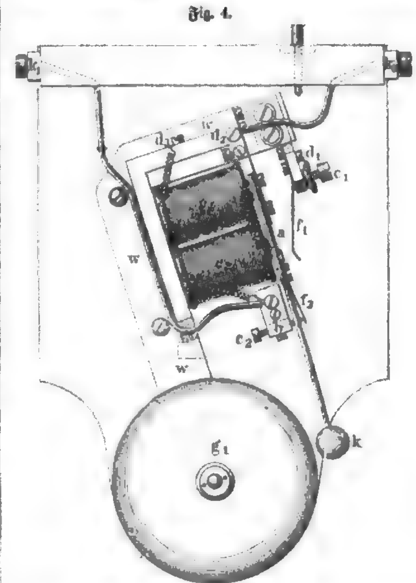
Klingel für Fernsprechtrommelbetrieb
