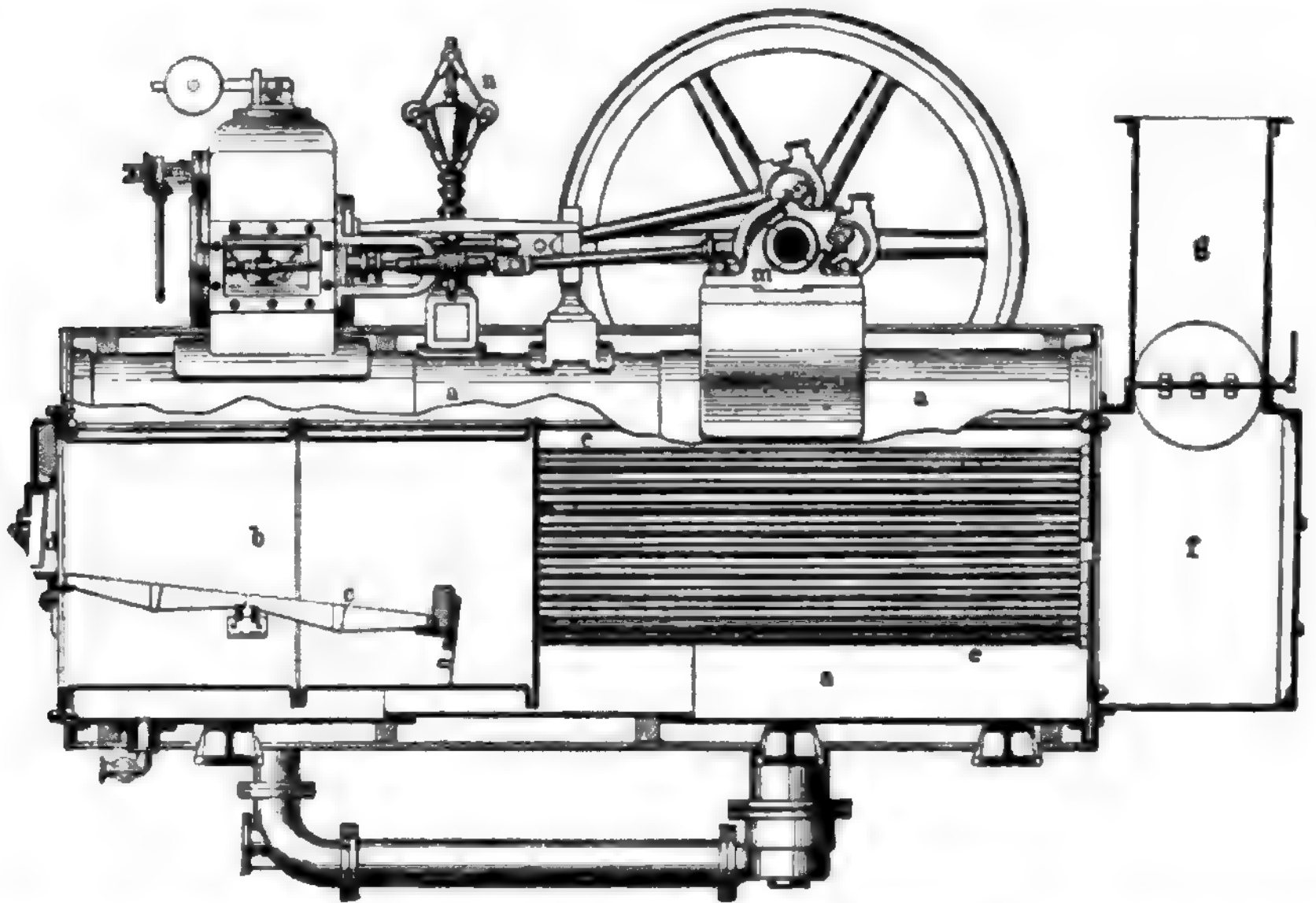
Halblocomobile mit Compoundmaschine. Längsschnitt.
