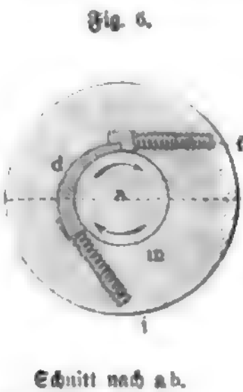
Kernaulsche Kuppelung
