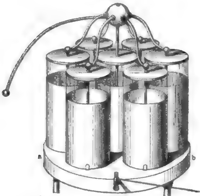
Batterie von Nieß.
