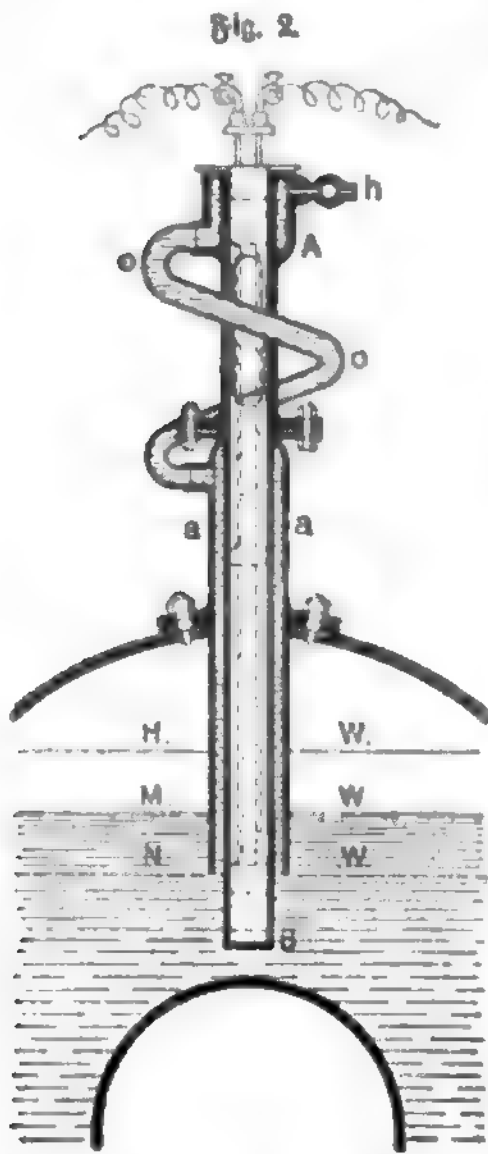
Schwarzkopff's Universalkontroll- und Sicherheitsapparat.
