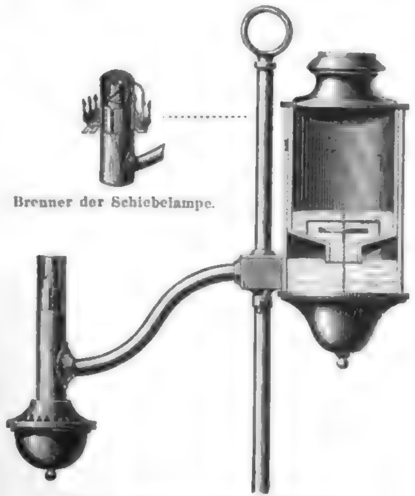
Fig. 2. Schiebelampe mit Sturzflasche.
