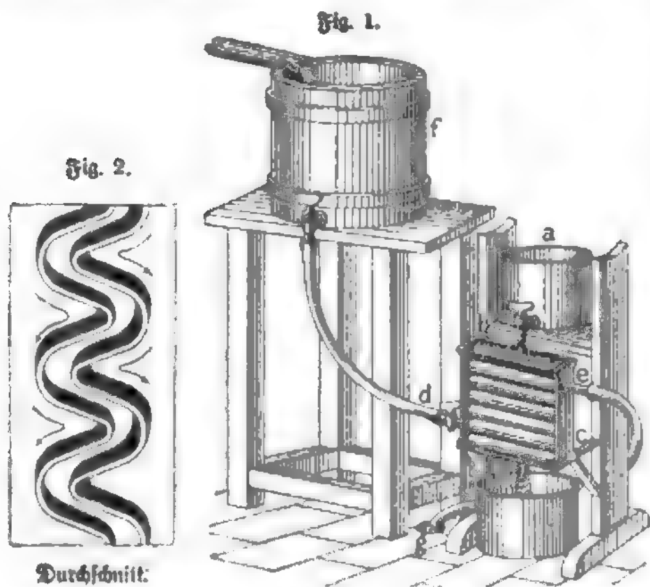
Fig. 1 u. 2. Lawrence'scher Kapillarkühler.
