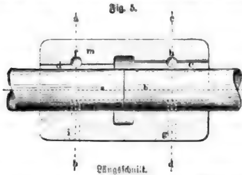
Kernaulsche Kuppelung
