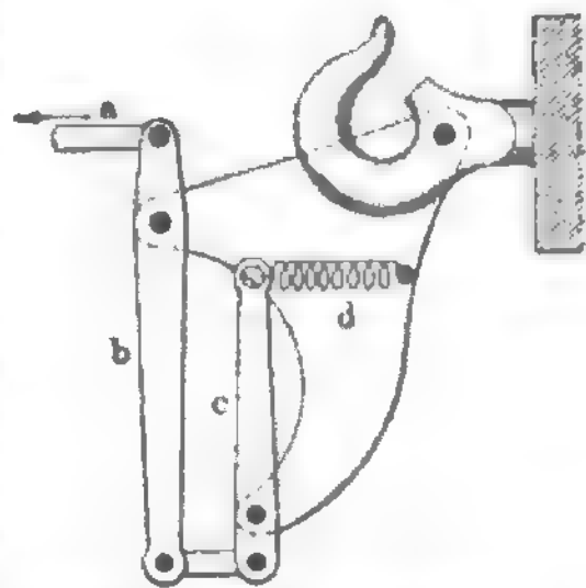
Kontrollapparat von Holz.
