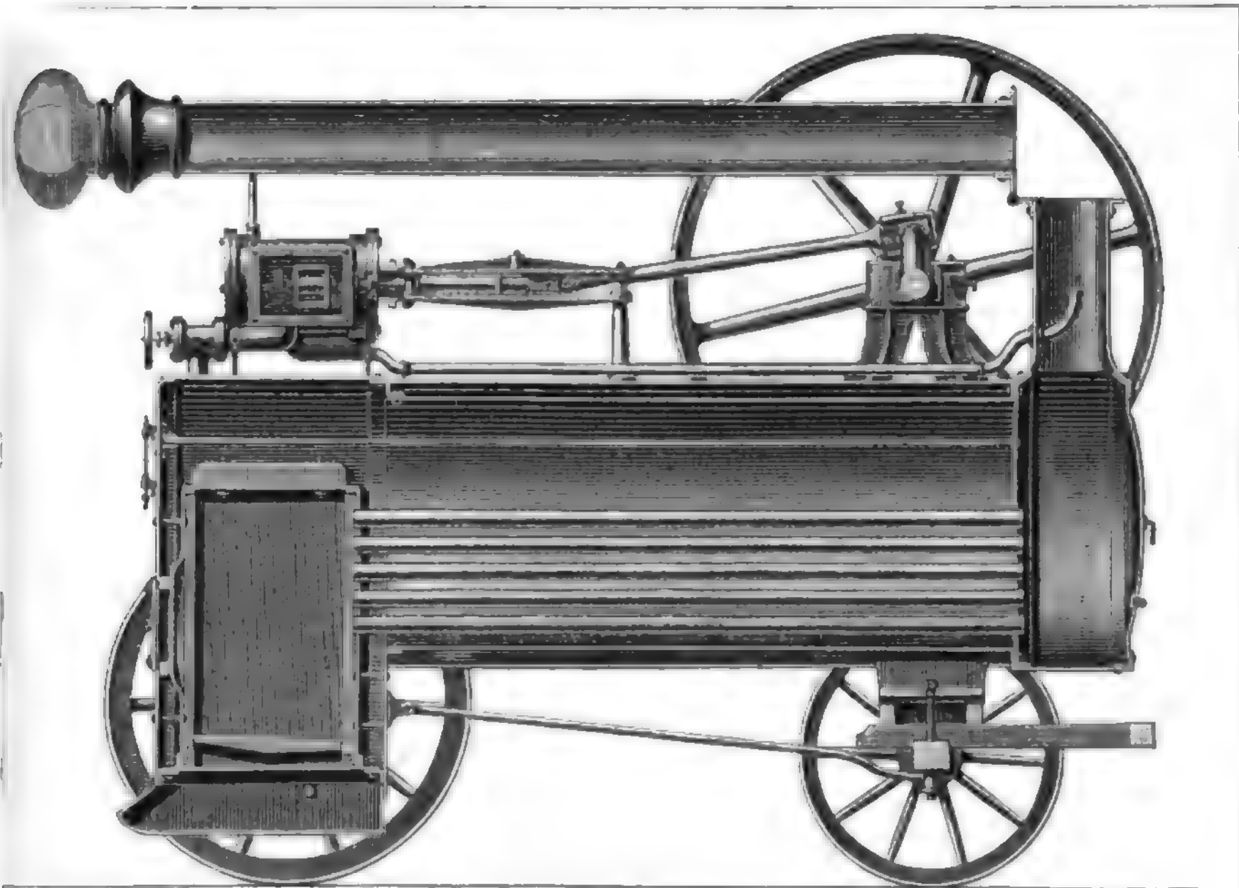
Fig. 2. Längenschnitt einer Lokomobile.
