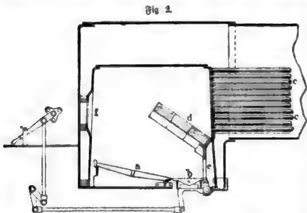
Repillische Feuerung. Längsschnitt.
