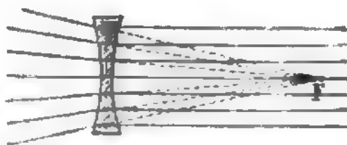
Virtueller Brennpunkt einer konkaven Linse.
