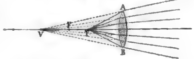
Konjugierte Punkte. (Virtueller Bildpunkt.)
