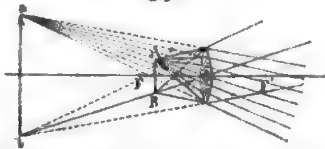
Virtuelles Bild durch eine konvexe Linse.
