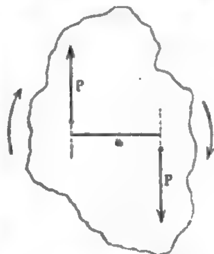
Kräftepaar.
