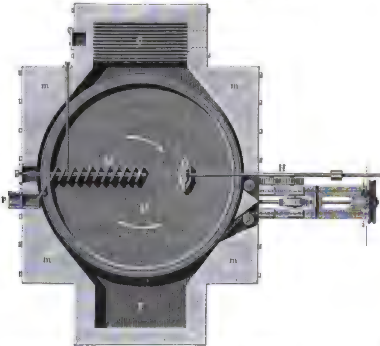
Fig. 5. Tellerofen von Gibb und Geislarp. Querdurchschnitt
