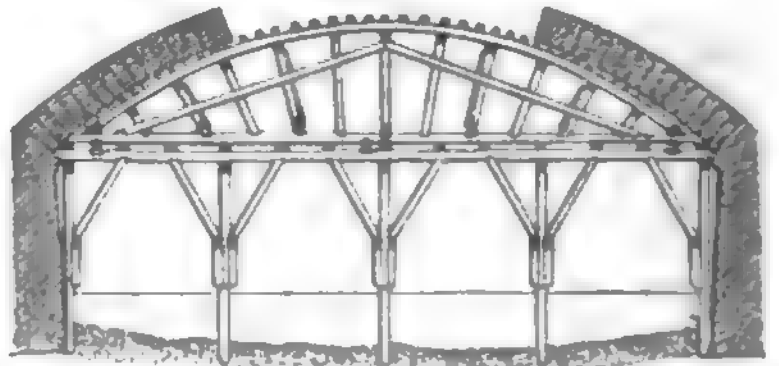
Stehendes Lehrgerüst.
