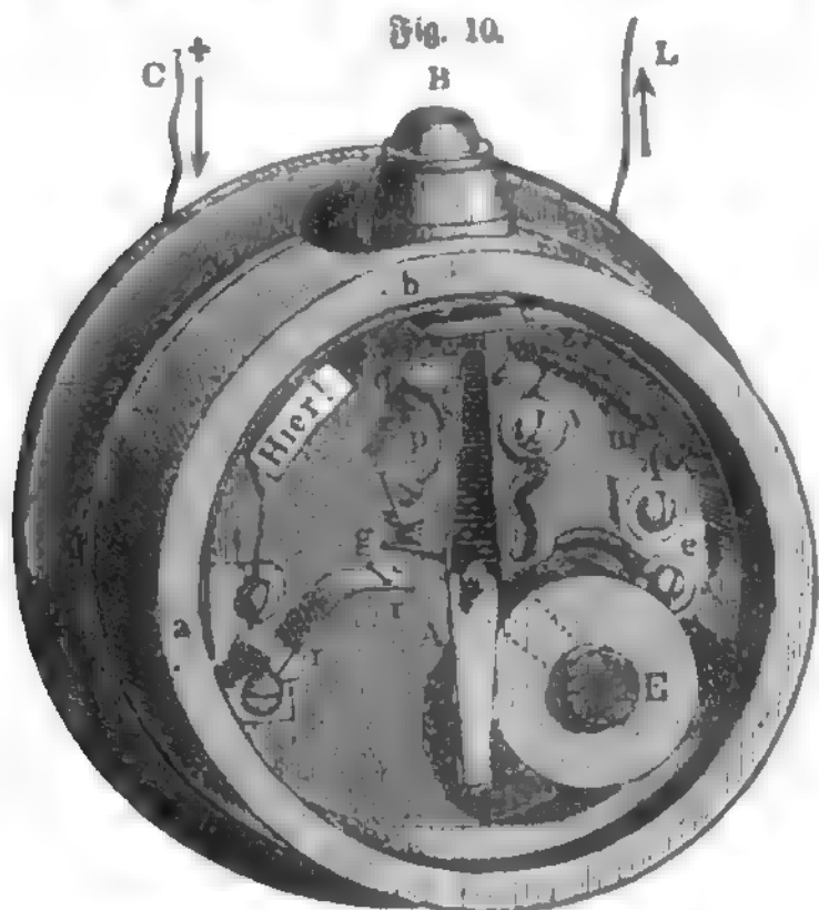
Elektrische Taste mit sichtbarem Rücksignal
