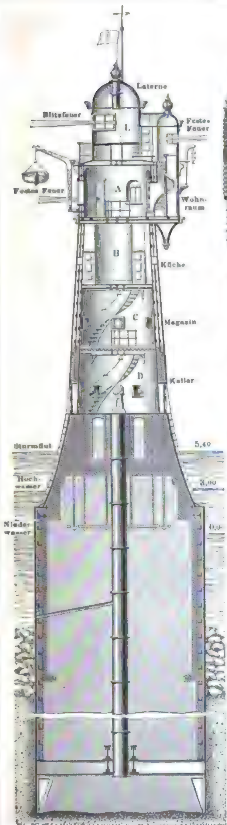
Fig. 1. Leuchtturm auf Rotersand. (Vertikalschnitt.)
