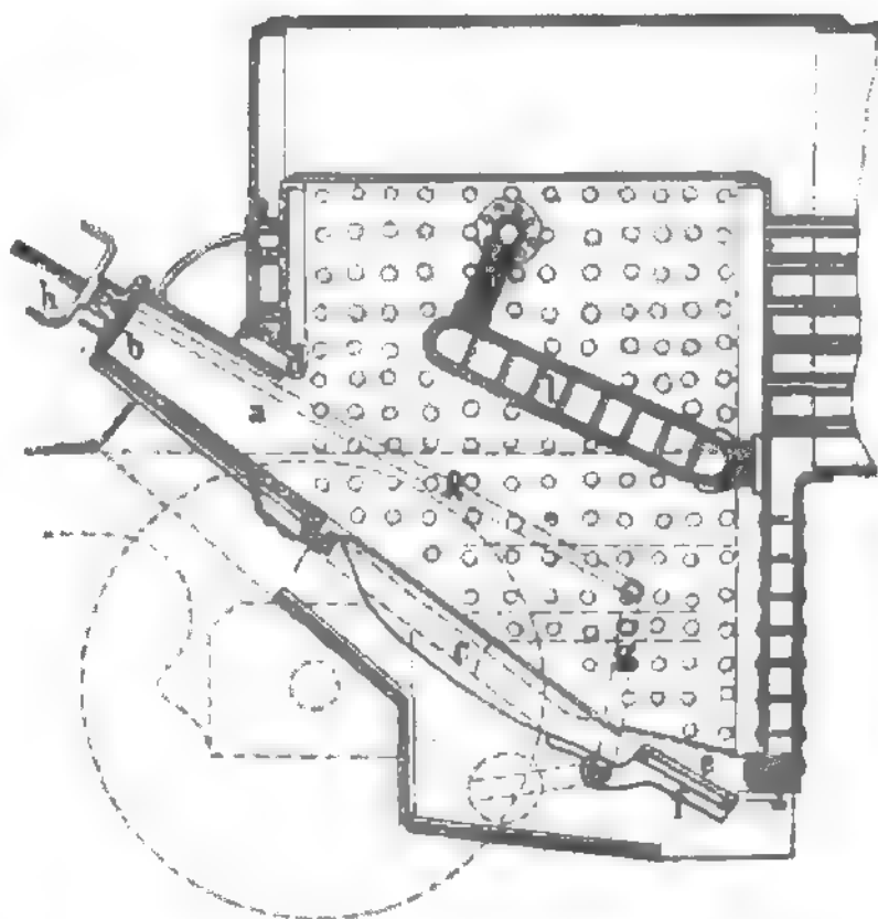
Tenbrink'sche Feuerung. Längsschnitt.
