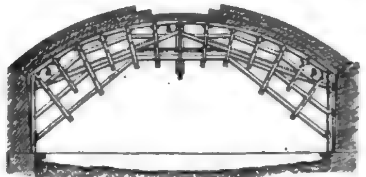
Gesprengtes Lehrgerüst.
