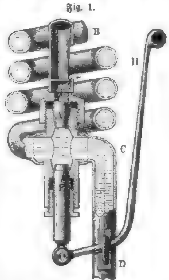
Blakes Alarmapparat.
