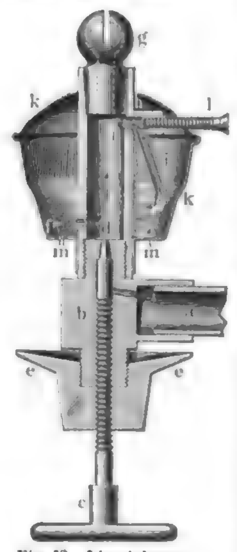
Fig. 12. Ligroinlampe von Bohm u. Brüder.
