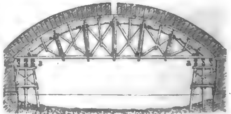
Lehrgerüst mit Fachwerkträgern.
