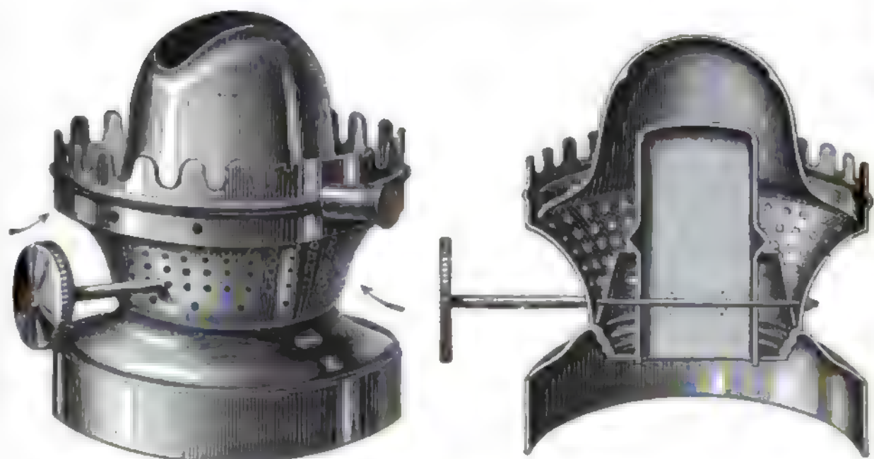
Fig. 4. u. 5. Flachbrenner für Petroleumlampen.
