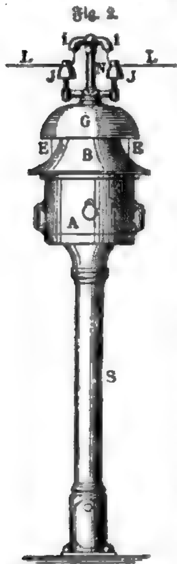
Spindelläutwerk von Siemens u. Halske
