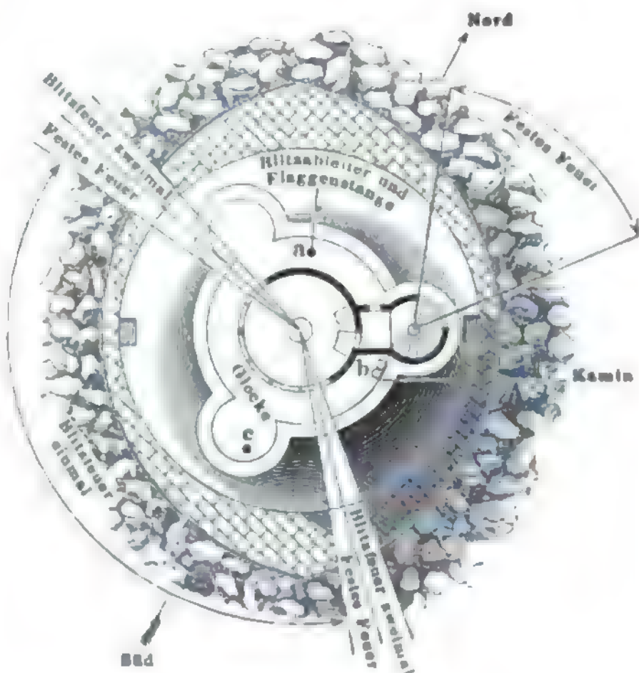
Fig. 2. Leuchtturm auf Rotersand. (Grundriß.)
