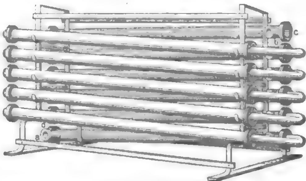
Rägell'scher Rühlapparat.
