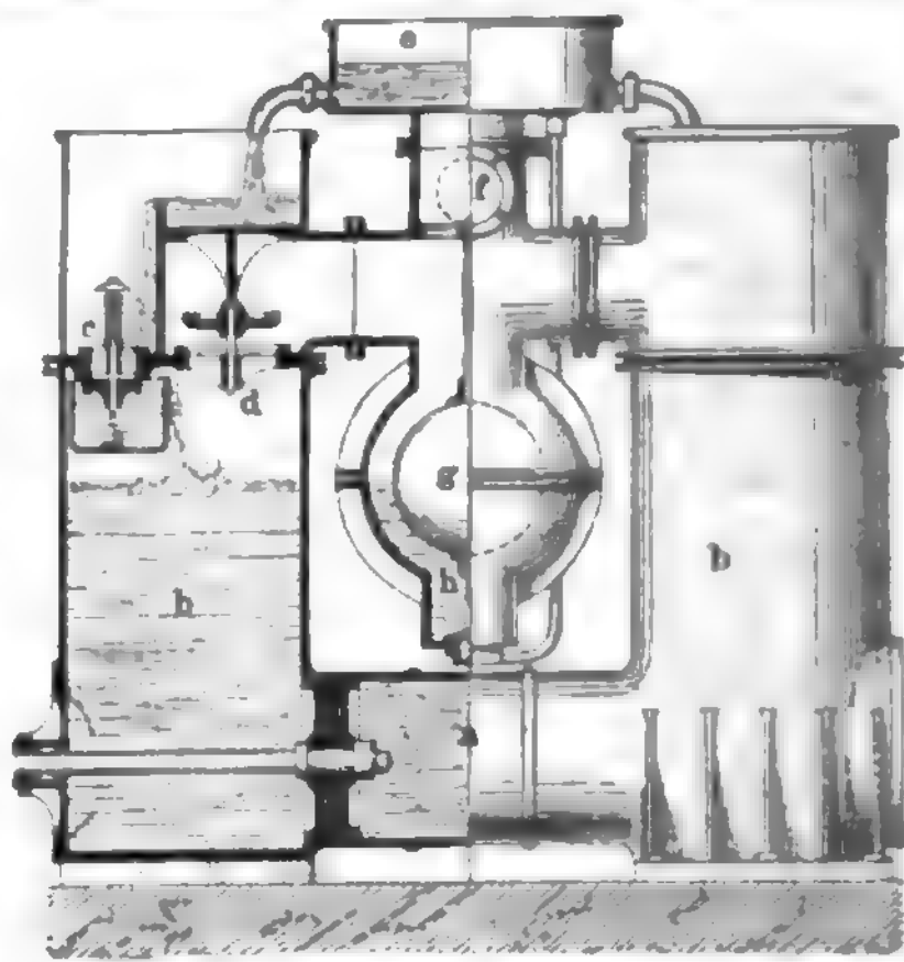
Fig. 1. Johnsons Luftverdichtungsmaschine.
