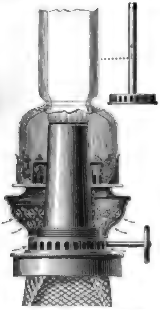
Fig. 8. Patent-Reformkosmosbrenner.
