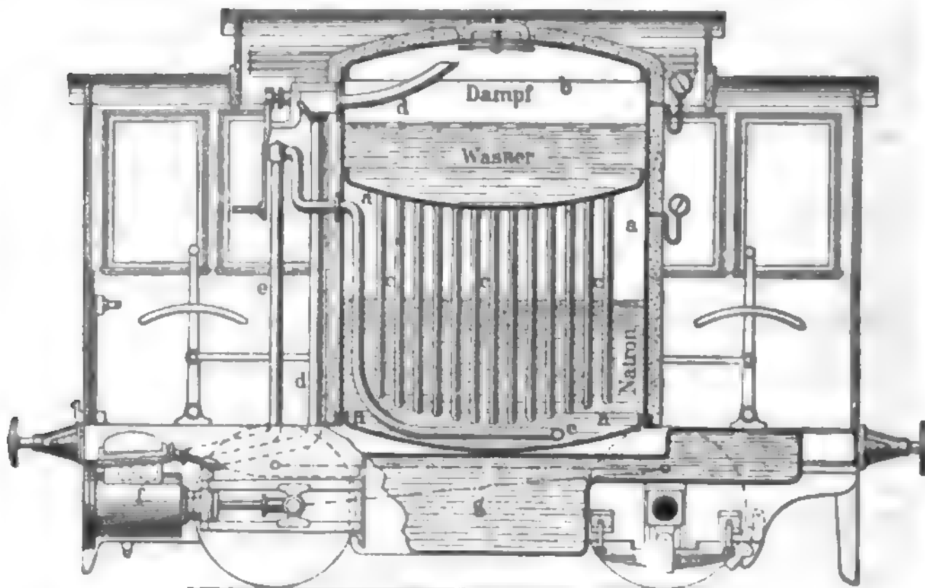
Honigmanns Natriumlokomotive. Bängschalt.
