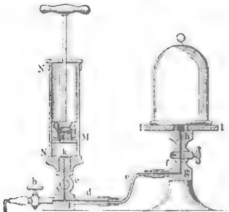
Fig. 1. Handluftpumpe.
