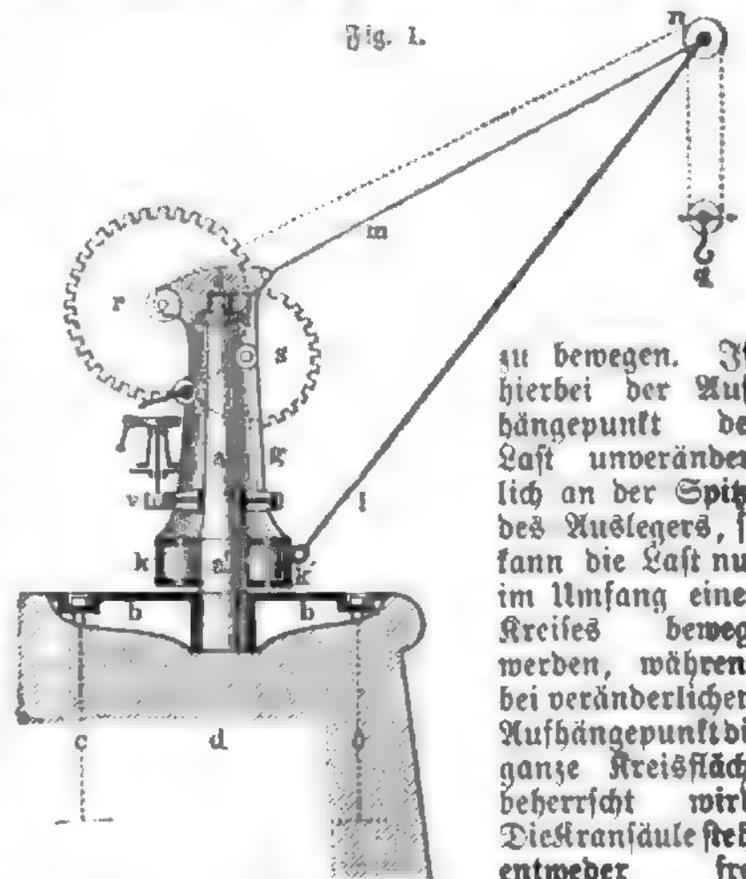
Frei stehender Kran. Uferkran.
