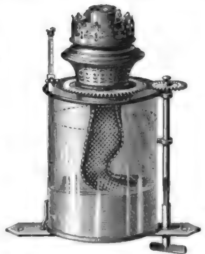
Fig. 6. Lampe mit begrenzter Brennzeit.
