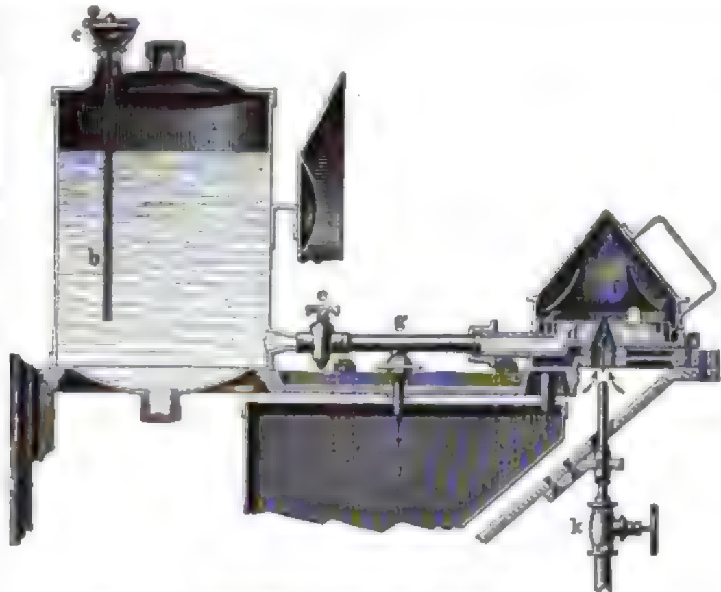
Fig. 13. Dampfstrahlampe für schwere Mineralöle.
