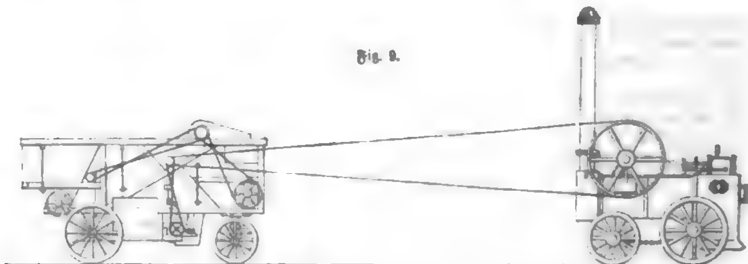
Betrieb einer Dreschmaschine durch die Lokomobile.
