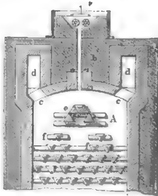
Gerstenhöfischer Ofen.
