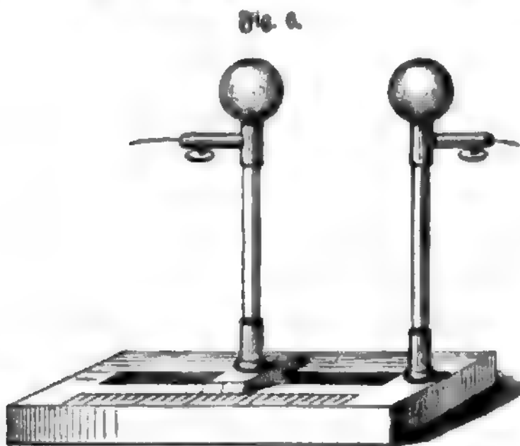
Funkenmikrometer.
