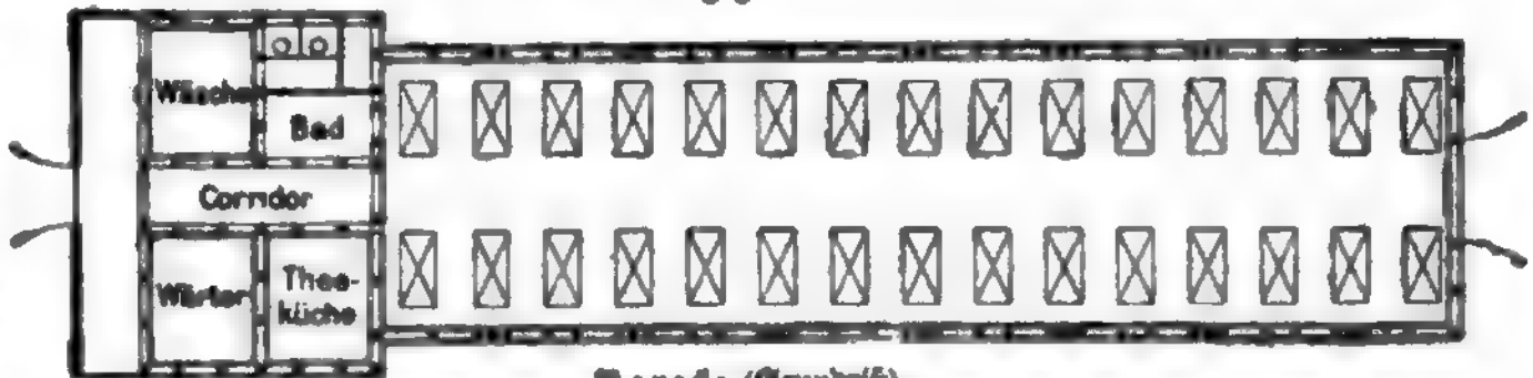
Baracke (Grundriß).
