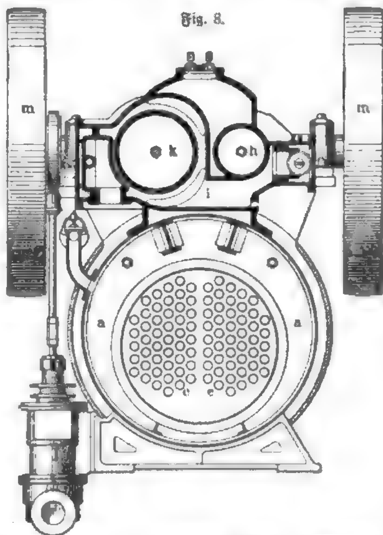
Halblokomobile mit Compoundmaschine. Querschnitt.
