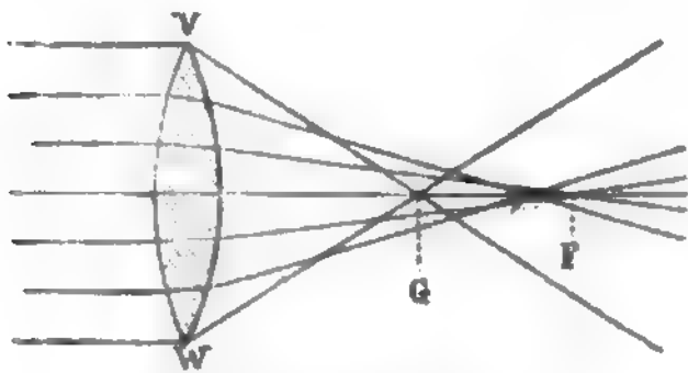
Sphärische Aberration.
