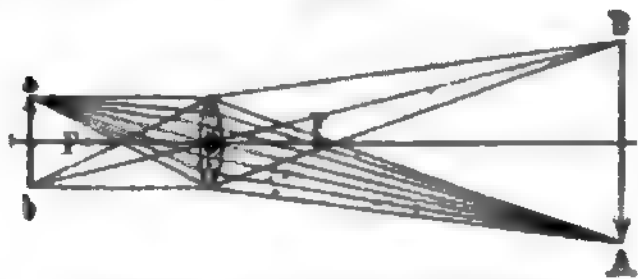
Entstehung eines reellen Bildes.
