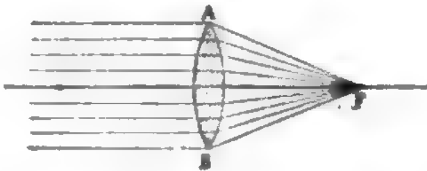
Brennpunkt einer konvergen Linse.
