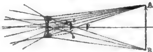
Virtuelles Bild durch eine konkave Linse.
