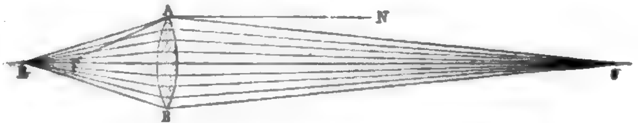
Konjugierte Punkte. (Reeller Bildpunkt.)
