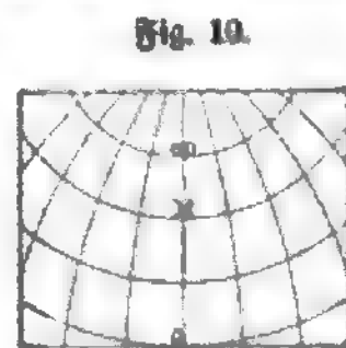
Bonnesche Projektion.
