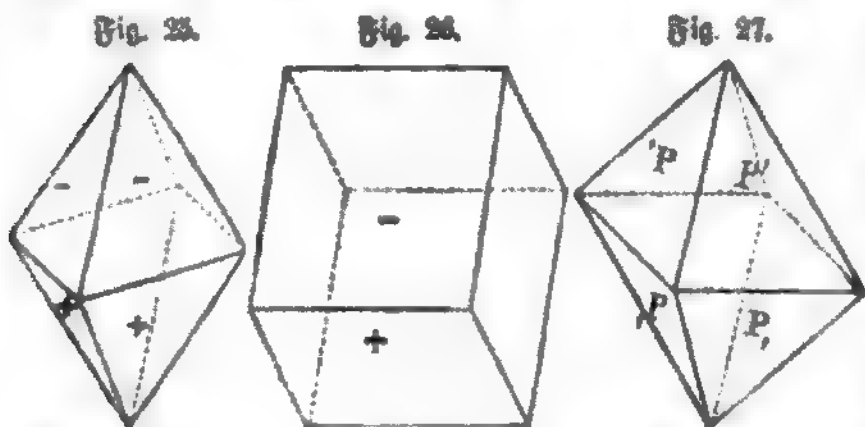
Monokline Pyramide Orthodoma Trikline Pyramide. Kristallformen des monoklinen u. triklinen Systems.
