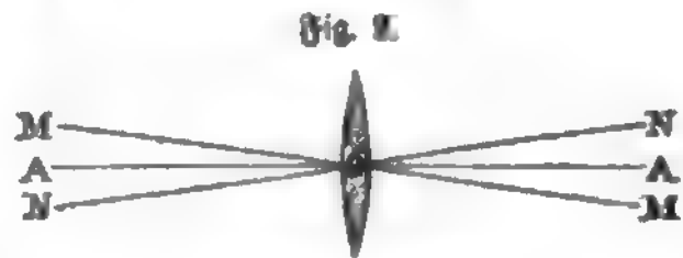
Achsen einer Linse.
