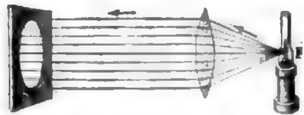
Ausstellt paralleler Strahlen aus einer bikonvexen Linse.
