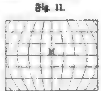
Flamsteedsche Projektion.
