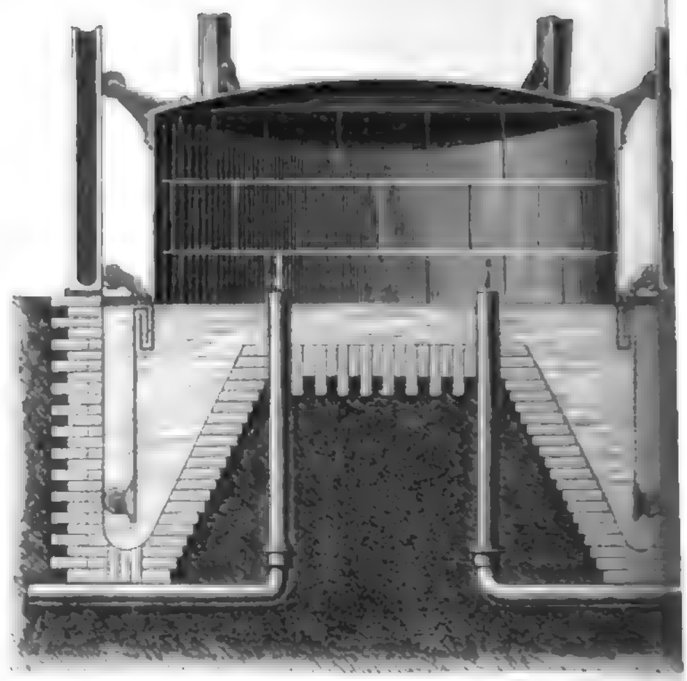
Fig. 7. Gasometer, Durchschnitt.
