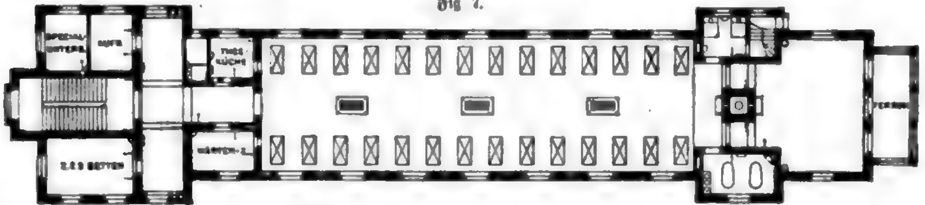
Zweistöziger Pavillon des Städtischen Krankenhauses in Berlin (Friedrichshain). Grundriß, Erdgeschoß.
