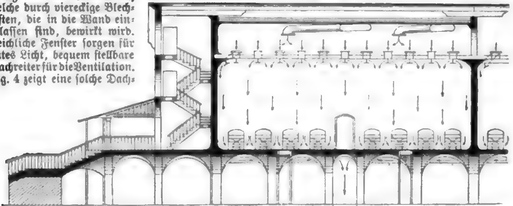
Isolierpavillon mit Unterbau und Dachventilation.
