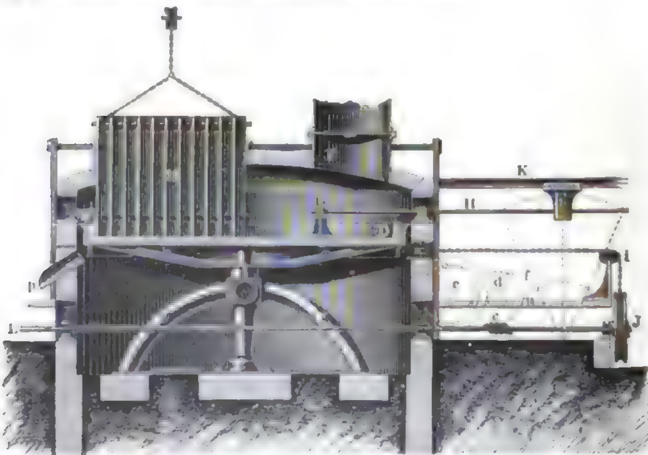
Fig. 4. Tellerofen von Gibb und Geislarp. Längsdurchschnitt.
