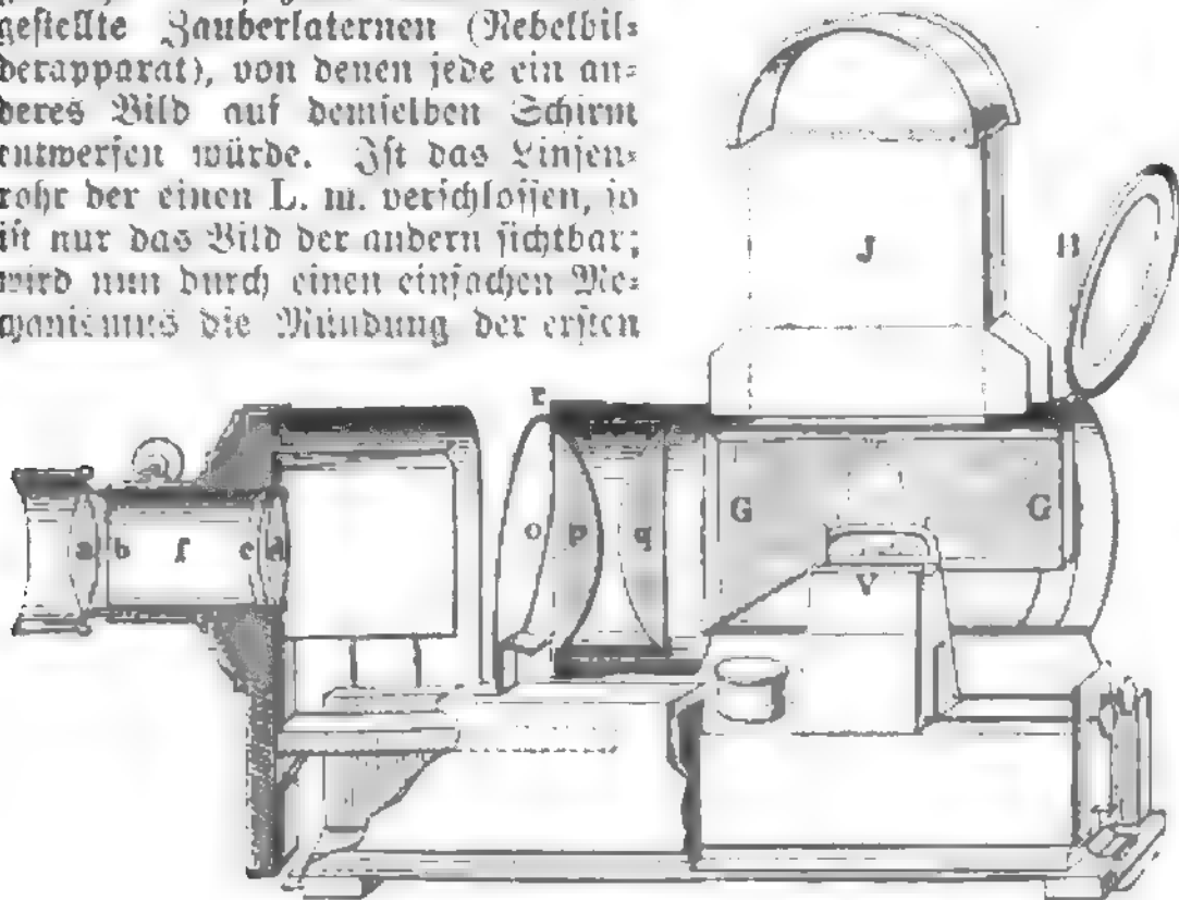
Erioptikon.
