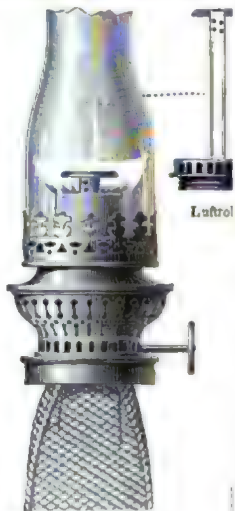
Fig. 7. Patentbrenner für Solaröl.
