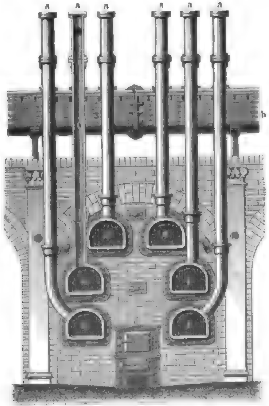
Fig. 1. Retortenofen, Vorderansicht.
