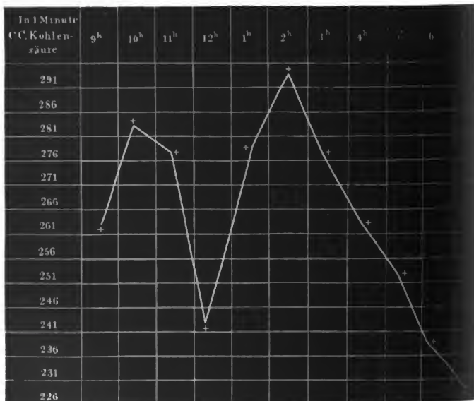
Fig. 2. Ausgeathmete Kohlensäure in einer Minute.
