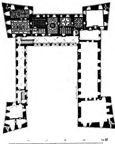
Obr. 110. Nelahoševy. Zámek. I. patro.
