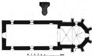
Obr. 93. Libušín. Půdorys kostela. Řez zebrá.
