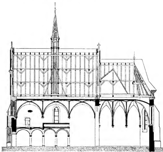
Obr. 265. Velvary. Rez děkaného kostela sv. Kateřiny.
