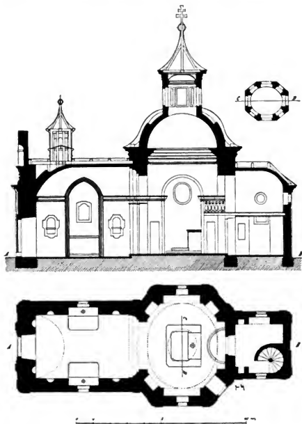
Obr. 146. Parlének. Půdorys a podélný řez kaple sv. Jana Nep.
