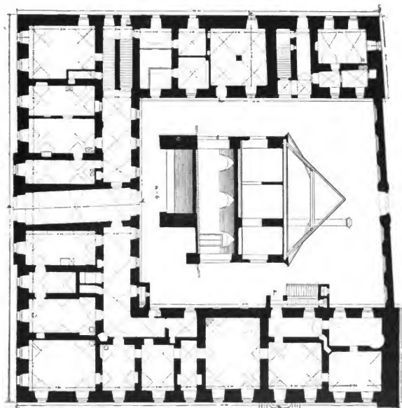
Obr. 104. Mětec. Půdorys a řez zámku.
