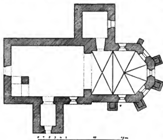
Obr. 41. Hostiář. Půdorys farního kostela.
