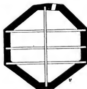
Obr. 95. Libuřín. Půdorys dřevěné zvonice.
