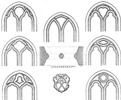
Obr. 276. Velvary. Kružba oken kostela sv. Jiří; domovní značka Jiřího Pechara.
