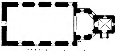
Obr. 245. Tuřany. Půdorys farního kostela.
