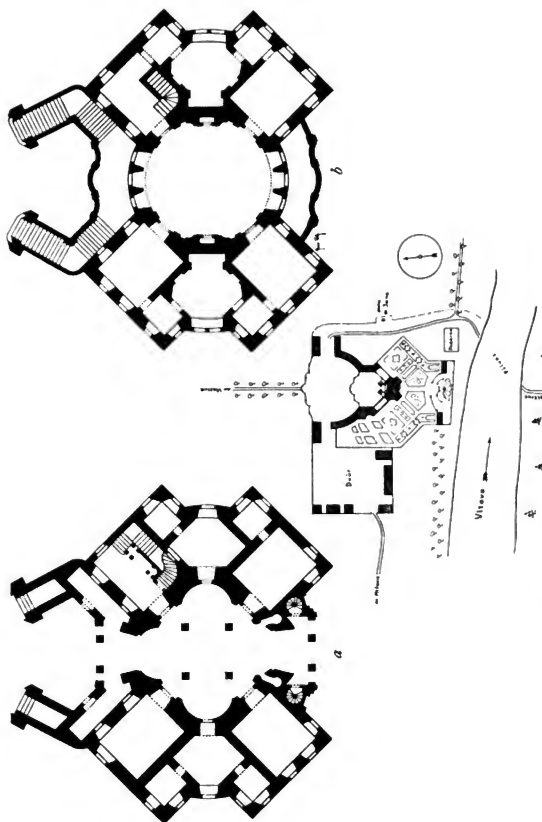
Obr. 247. Veitruvy. Zámek. Situační plán z r. 1744. a) přilehlí. b) I. patro.
