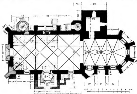
Obr. 256. Velvary. Půdorys děkanského kostela sv. Kateřiny.
