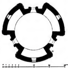
Obr. 53. Hostiář. Půdorys hřbitovní kaple.
