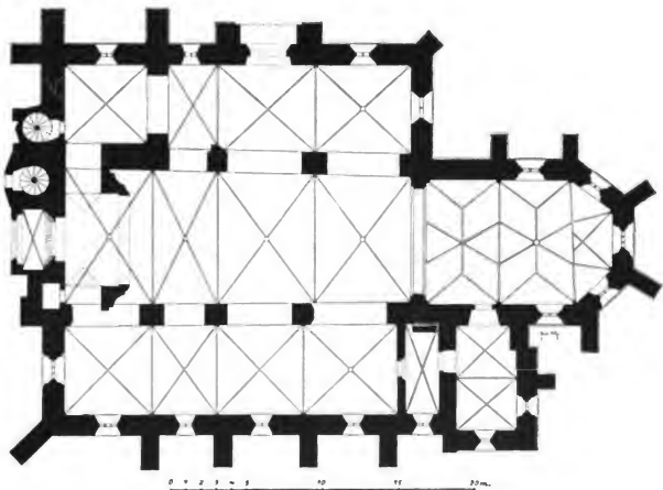
Obr. 172. Půdorys děkanského kostela.
