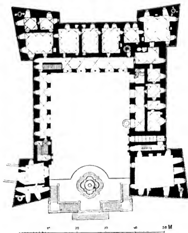
Obr. 106. Nelahozeves. Půdorys zámku.
