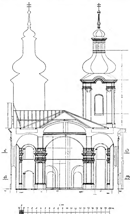
Obr. 292. Zionice. Příčný řez kostela; pohled k presbytěři.
