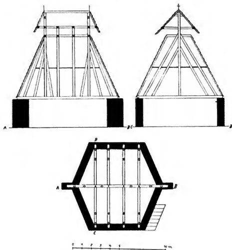
Obr. 83. Kvilice. Půdorys a řezy zvonce.
