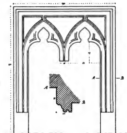
Obr. 48. Hostiář. Sedíle s průřezem.
