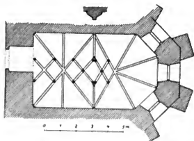
Obr. 207. Smečno. Zámecká kaple sv. Anny; profil šebra.
