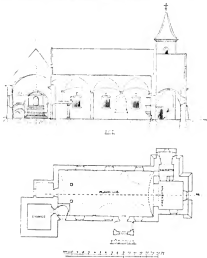
Obr. 248. Půdorys a řez farního kostela.
