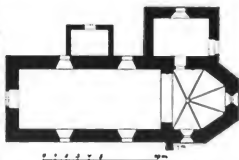
Obr. 304. Želenice, Půdorys kostela.
