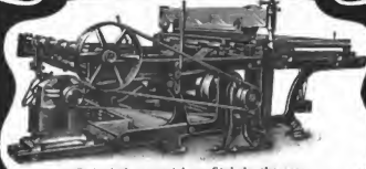
Elektrisch angetriebene Steindruckpresse.
