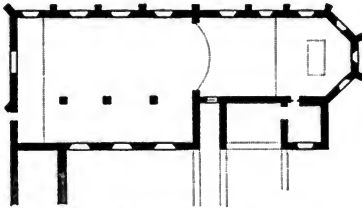
Grundriss der Marienkirche zu Weida 1:600 nach Walther, Das alte Weida.
