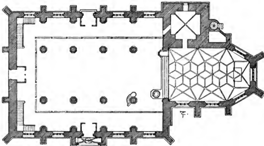
Grundriss der Johanniskirche zu Neustadt a. O. 1 : 400.
