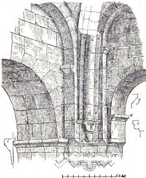
Gewölbe-Anfang in der Nordkapelle der Kirche zu Veitzberg nach einer Zeichnung von Herrn Baurath Dr. Mothes.
