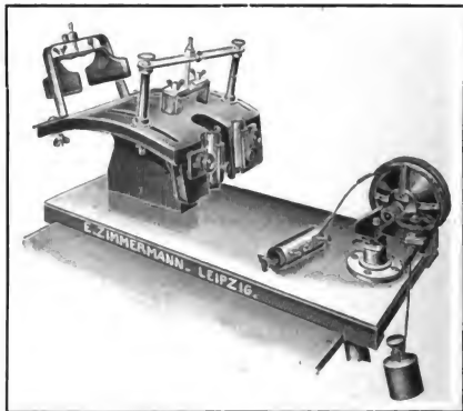
Fig. 5. Ergograph (nach Meumann).
