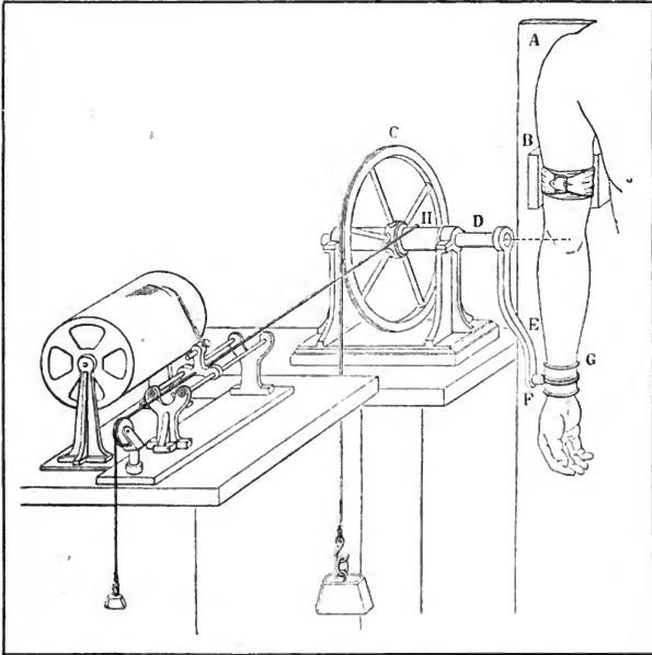
Fig. 3. Ergograph zur Untersuchung der Arbeitsleistung des Biceps. (Tréves, Le travail, la fatigue et l'effort . L'Année psychologique, 1906.)
