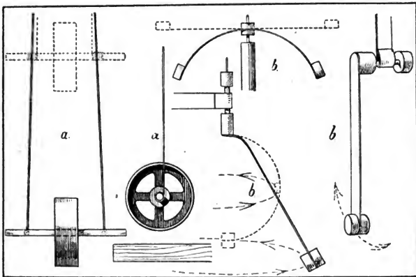
Fig. 5. a) Maxwell's Vertikalpendel als Fallmaschine. b) Achse fŕr Schwingversuche.
