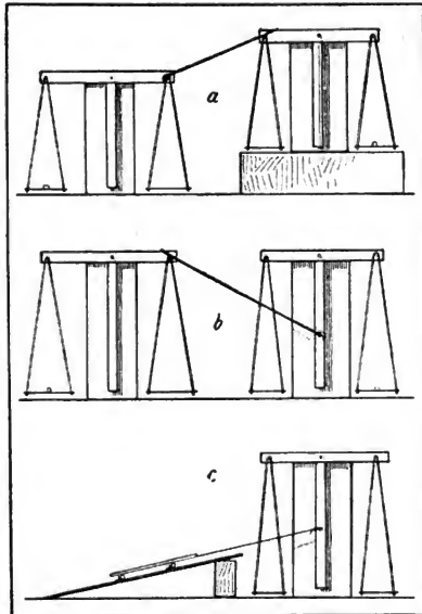
Fig. 3. a) Doppelwägung eines schrägliegenden Drahtes. b) Schubwirkung eines schrägliegenden Drahtes. c) Schiefe Ebene.
