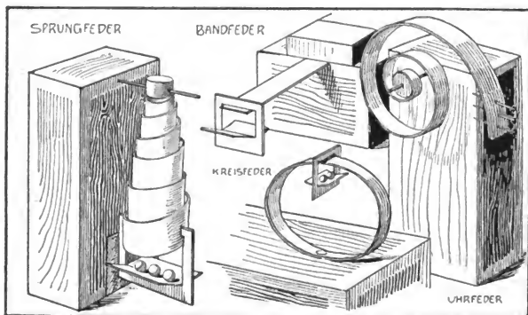
Fig. 6. Federn aus Papierstreifen.
