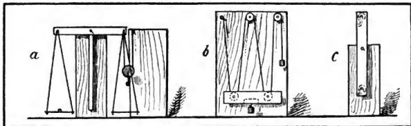
Fig. 4. a) Einfache Seilfleyscheibe (lose Rolle). b) Doppelte Seilfleyscheibe (Flaschenzug). c) Doppelpendel.
