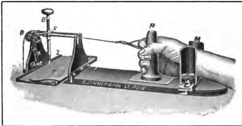
Fig. 6. Ergograph (nach Dubois).
