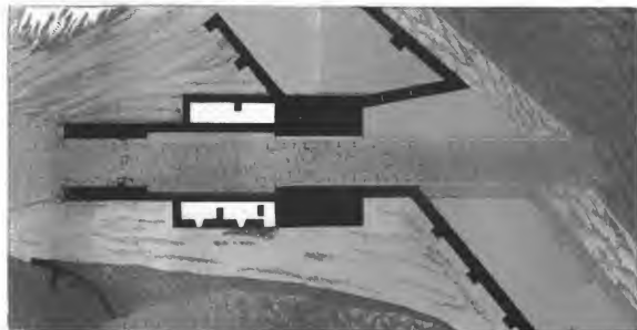
Fig. 15. Grundriß des nolaner Thors.
