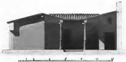
Fig. 147. Restaurirter Durchschnitt desselben auf der Linie a—b .
