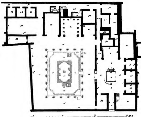
Fig. 167. Plan der Casa di Meleagro.
