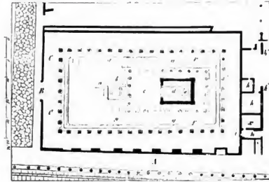
Fig. 57. Plan des s. g. Venustempels.
