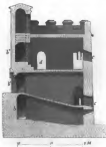
Fig. 13. Durchschnitt eines Thurms.
