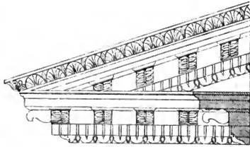
Fig. 266. Giebel mit abgeschrägten Kragsteinen.
