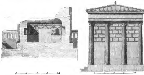
Fig. 222. Durchschnitt und Restauration des großen Grabmals.
