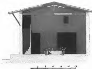
Fig. 152. Restaurirter Durchschnitt auf der Linie a—b .
