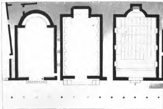
Fig. 77. Plan der s. g. Curien oder Tribunalien.
