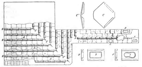
Fig. 139. Dach im Peristyl der Casa di Sirico .
