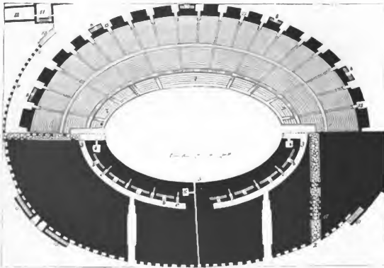
Fig. 101. Plan des Amphitheatere.
