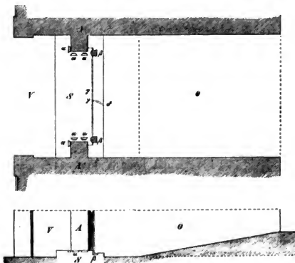
Fig. 134. Hausflur der Casa di Pansa.
