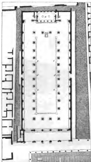
Fig. 79. Plan der Basilika.
