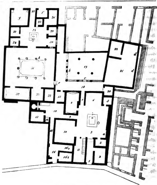
Fig. 170. Plan des Hauses des Siricus.
