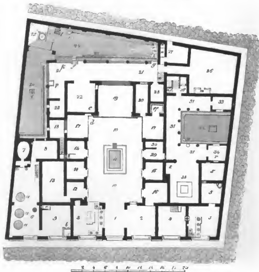
Fig. 165. Plan der Casa di Sallustio.
