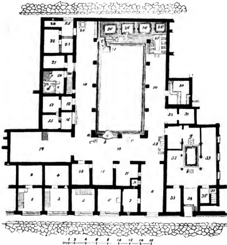
Fig. 192. Plan der Fullonica.
