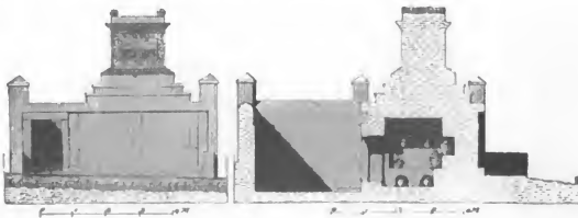
Fig. 204. Grab der Naevoleia Tyche. Ansicht und Durchschnitt.
