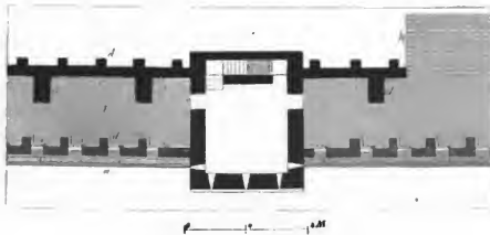
Fig. 6. Grundriß der Mauern.
