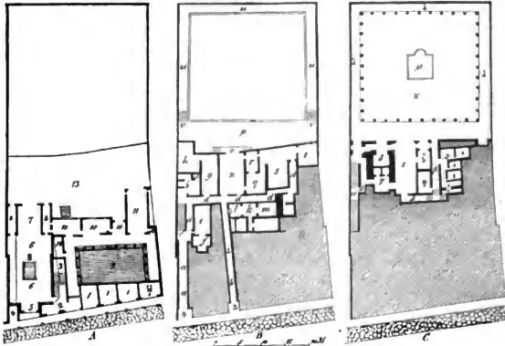
Fig. 178. Plan eines dreistöckigen Hauses.
