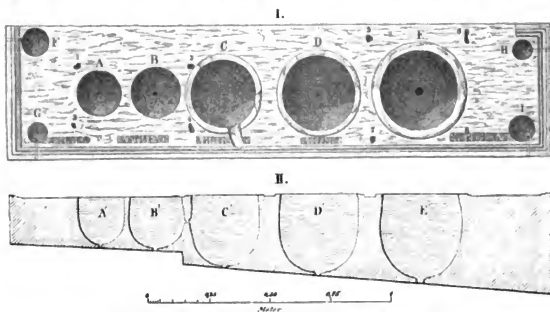
Fig. 29. Ansicht und Durchschnitt des Maßtisches.
