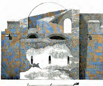
Fig. 11. Ansicht eines Thurmes.
