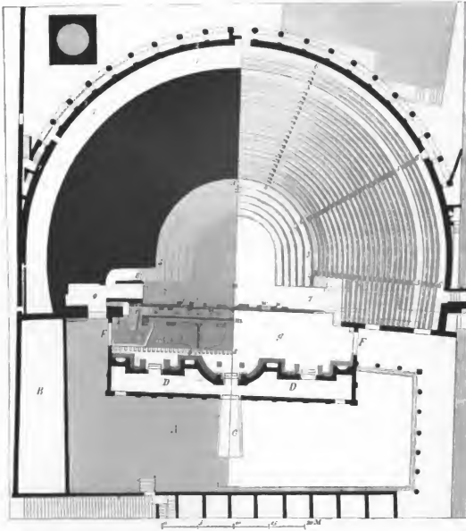
Fig. 86. Plan des großen Theaters.
