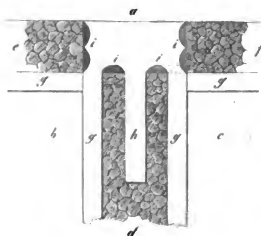
Fig. 21. Plan eines Emissars.
