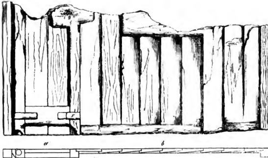
Fig. 183. Plan und Ansicht eines Ladenverschlusses.
