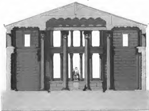
Fig. 52. Restaurirter Durchschnitt der Basilika (nach Mazois).
