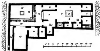
Fig. 153. Plan der Casa della toilette dell' Ermafrodito.
