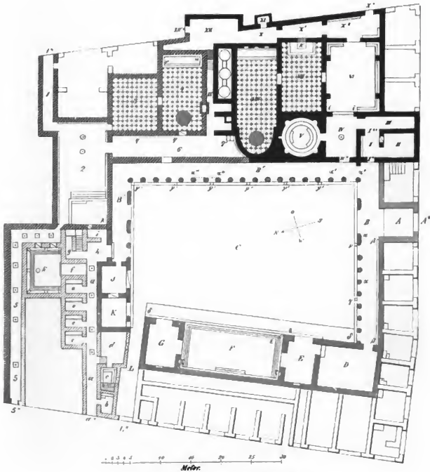
Fig. 123. Plan der größeren Thermen.
