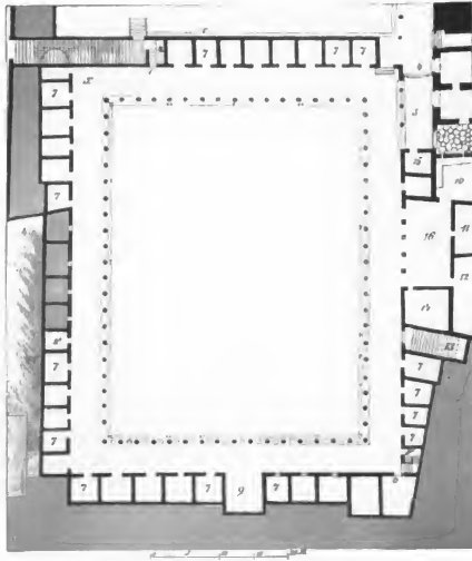
Fig. 113. Plan der Gladiatorencaserne.
