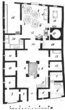
Fig. 188. Plan einer Bäckerei.
