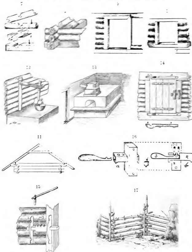
Fig. 7—17. 7 und 8 Verzäpfung beim Rundholzbau. 9 Türstock. 10 Fensterstock. 11 Dachstuhlkonstruktion. 12 Kesselhälter. 13 Heiz-, Koch- und Backofen. 14 Haustür mit Holzbindern und Holzriegel. 15 Einfaches offenes Holzschloß. 16 „Blindes“ Holzschloß ( a Ansicht, b Durchschnitt): B Schloßbalken, S Schlüssel, mit dem die Fallhölzchen ii gehoben werden, welche den Riegel R festhalten. 17 Zaun.
