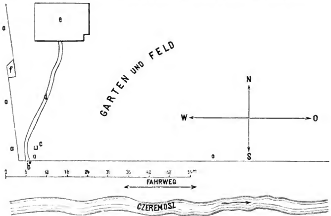
Fig. 3. Situationsplan eines mittelgroßen buzulischen Gehöftes in Uscieryki am Czeremoszflusse (Galizien). aaaa Zaun aus Holzstangen (vgl. Fig. 17); derselbe läßt sich an jeder beliebigen Stelle leicht auseinandernehmen, um mit dem Wagen hereinfahren oder Vieh durchtreiben zu können. b Durchlaßtor aus Stangen, die in den Torsäulen verschiebbar angebracht sind; diese letzteren sind zum Schutze gegen die Feuchtigkeit oben mit Setzplatten bedeckt; die oberste verschiebbare Stange ist gewöhnlich herabgenommen, damit Fußgeher das Tor übersteigen können; zu diesem Zwecke liegt neben denselben auch ein Stein (vgl. Fig. 18). c Brunnen. d Steg zum Hause. e Haus (vergleiche die folgenden Figuren). f Schweinestall.
