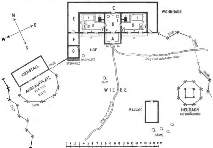
Fig. 1. Grundriß eines großen buzulischen Gehöftes in Kosmacz (Galizien, Bezirk Kossów). A Gang, B Vorhaus, C und D Stube, EE Winterstallungen und Aufbewahrungsort für allerlei Fässer und Geräte, F überdeckter Raum, gegen den Hof ganz offen, G ein kleiner Stall, aa Ofen, bb Bettgestelle, cccc feststehende Bänke, d Kiste, e Tisch, ff Geschirrkasten, bei g hängt an der Wand ein Wandbrett und neben demselben Bilder, ein Dreilicht, Töpfchen, Blumen, Handschuhe u. dgl., h eine tragbare Bank, ii zwei Stühle, bei k der Hackenhälter, ll große Fässer, bei mm sind Eisenringe befestigt, an denen die Reitpferde angebunden werden, nn Vorbänke beim Hause. Die Stube links hat Fensterläden. Man vergleiche die folgende Figur, welche den in demselben Maßstabe gefertigten Grundriß des Nachbarhauses zeigt, zu dem der nach rechts ziehende Steg führt und das einem armen Manne gehört.
