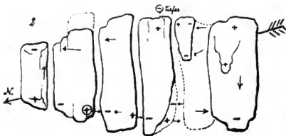
Fig. 2. Grundriß (Skizze) eines Magnetsteinfelsens an der gleichen Stelle wie obiger Fels, 33 Schritte südwestl. vom Signal, der Pfeil gibt immer die Richtung der Nordnadel an, die Pole im Ring liegen etwas unter der Oberfläche. Die punktierten Teile der Felsen liegen tiefer, sind meist von Moos bedeckt, und heben sich nicht scharf ab. Die ganze Länge der Felsparthie beträgt gegen 2 m, die Breite durchschnittlich 0,70—0,80 m. (Skizzirt 1887.)
