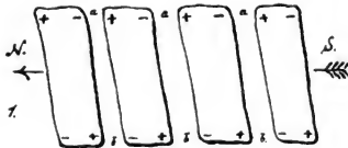
Fig. 1. Grundriß eines zerklüfteten Magnetsteines v. Frankenstein südlich vom Signal, ab Klüfte. Copie nach Ludwig und Seibert, 1863
