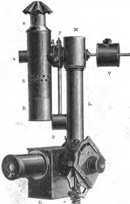
Fig. 18. v. Gothard's Pointer-Ocularkopf in Ansicht.
