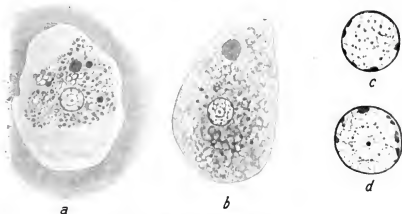
Fig. 1. Entamoeba tetragena .
