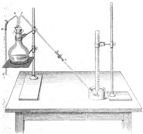
Apparat zur Salpetersäurebestimmung nach Schulze - Tiemann
