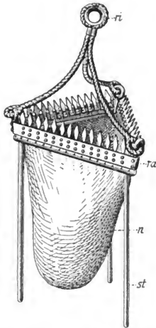
Fig. 615. Dredsche n. REINKE. ra Rahmen, n Netz, ri Ring, st Stäbe.
