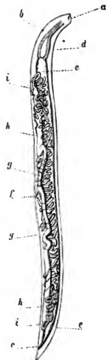
Dochmius duodenalis fem. Geschlechtsorgane.
