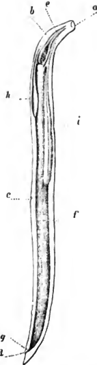
Dochmius duodenalis fem. Darmtractus.
