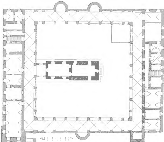
Obr. 26. Hájecký klášter s kaplí P. Marie. Půdorys
