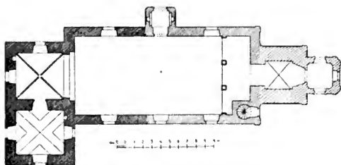
Obr. 15. Družec. Kostel P. Marie. Půdorys.
