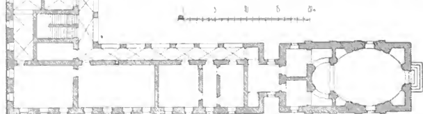
Obr. 5. Buřtůvhrad. Půdorys zámku před přístavbou kaple.
