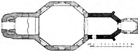
Obr. 97. Tachlovice. Kostel sv. Jakuba. Půdorys.
