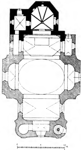
Obr. 44. Nezdice Dolní. Kostel sv. Prokopa. Půdorys.
