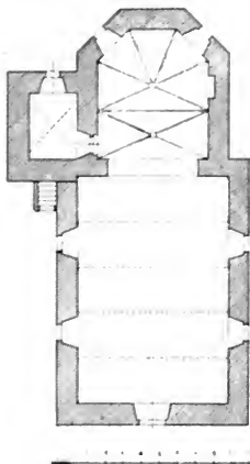
Obr. 2. Buková. Kostel sv. Jiří. Půdorys.
