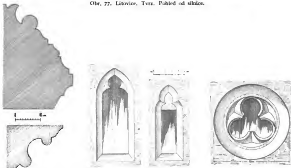
Obr. 78.—80. Litovice. Tvrz. Ostění okén v 2. patře na severu (nahore) a na jihu (dole). Okénka v jižním schodišti. Okénko v arkýři.
