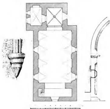
Obr. 46. Petrovice. Kostel sv. Vojtěcha. Pádorys a detaily.
