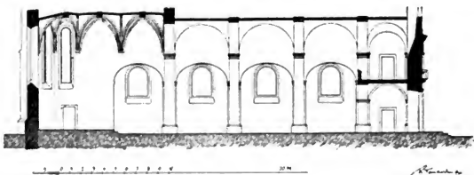
Obr. 84. Zelená Hora, Kostel P. Marie, Podélný řez.
