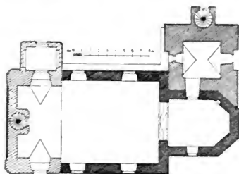
Obr. 106. Unhošt. Kostel sv. Petra a Pavla. Püders.
