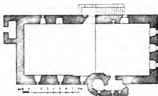
Obr. 75. Litovice, Půdorys tvrze.
