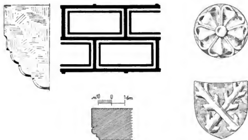
Obr. 1. Buštěhrad. Zbytky hradu: krákoec, schema rustiky, profil schodního kamene a svorníky.
