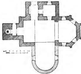
Obr. 89. Svárov. Kostel sv. Lukáše. Půdorys.
