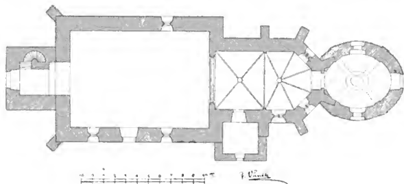
Obr. 6. Hořovice. Kostel sv. Matěje. Půdorys.
