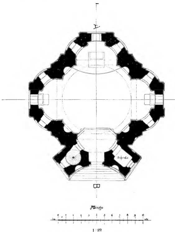
Obr. 59 Kladno, Kaple sv. Floriána, Půdorys.
