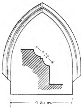
Obr. 25. Měčín, Kostel sv. Mikuláše. Sedle.
