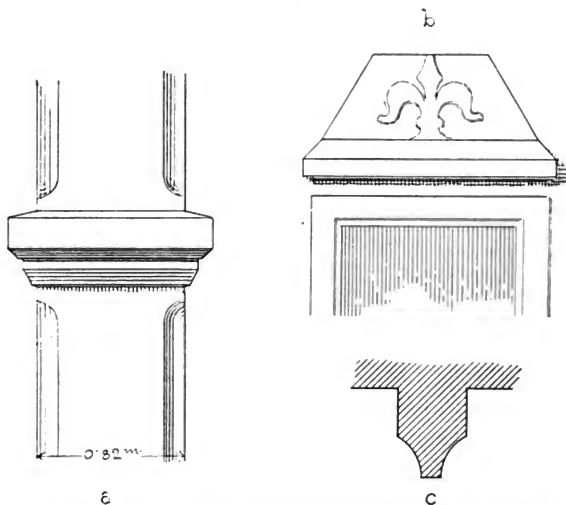
Obr. 65. Vleov, Kostel sv. Ambrože: a patka vítězného oblouku, b sanktuarium, c profil žebra
