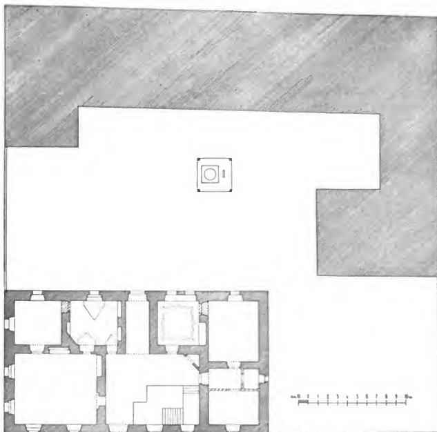
Obr. 100. Toskána. Půdorys domu s dvorem.
