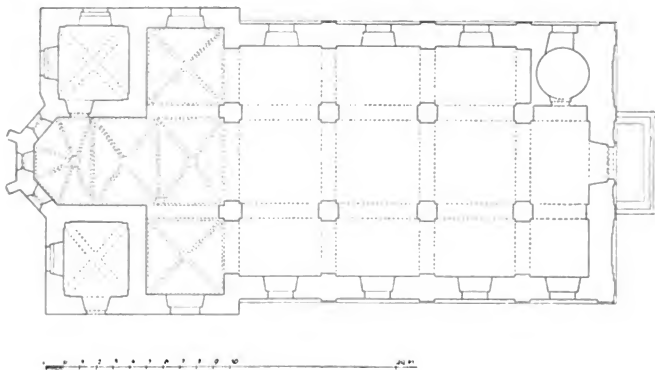
Obr. 83. Zelená Hora, Kostel P. Marie, Pádorys.
