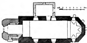
Obr. 114. Vřetovice. Kostel sv. Václava. Půdorys.
