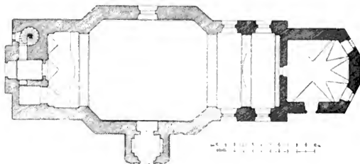
Obr. 70. Lidice. Kostel sv. Martina, Půdorys.
