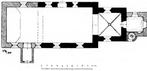
Obr. 49. Prádlo, Kostel Povýšení sv. Kříže, Pádras.
