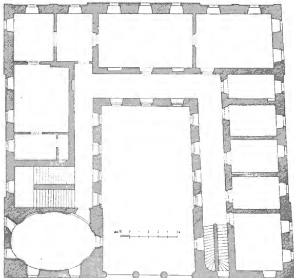
Obr. 62. Kladno. Půdorys zámku.
