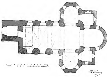
Obr. 27. Mileč, Kostel sv. Petra a Pavla, Pádorys
