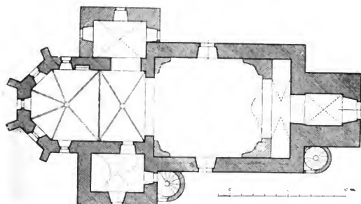
Obr. 24. Mečín, Kostel sv. Mikuláše, Půdorys.
