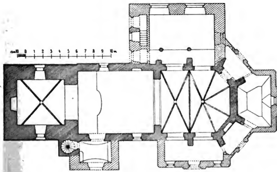
Obr. 42. Hostivice. Kostel sv. Jakuba. Půdorys.
