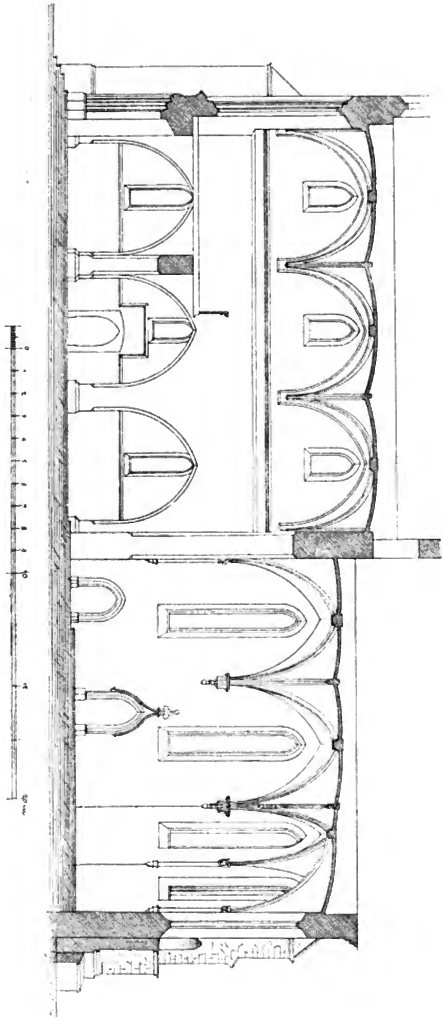
Obzr. 34. Nepomuk, Kostel sv. Jakuba, vnitřní řez.
