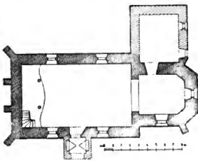
Obr. 117. Zelezná. Kostel P. Marie. Püderys.
