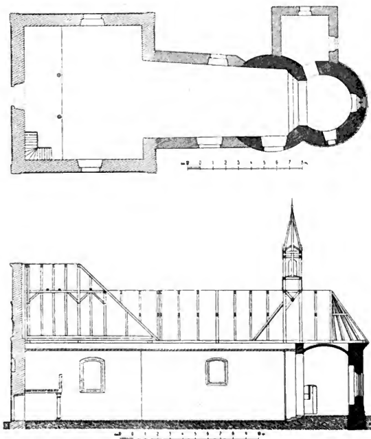
Obr. 84. a 85. Rapice. Kostel sv. Mikuláše. Půdorys a řez podélný.
