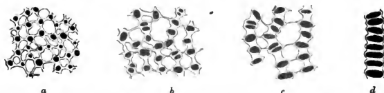
Figur 4. Schematische Darstellung der Bildung des Keratfadens aus dem Gerüst des ruhenden Kerns; die Nucleinkörner sind schwarz eingezeichnet; Vergr. e. c. 5000.
