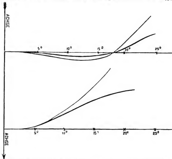
Bildfeld-Durchschnitt eines Petzval'schen Portrait-Objectivs.
