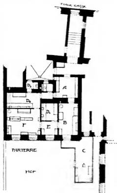
Fig. 57. Grundriss des Laboratoriums.
