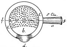
Fig. 8. Weißblechsieb zum Fangen der Culicidenlarven und Puppen, von oben. f bis g 15 cm. Durchmesser des Siebbodens (c b) 8 cm.
