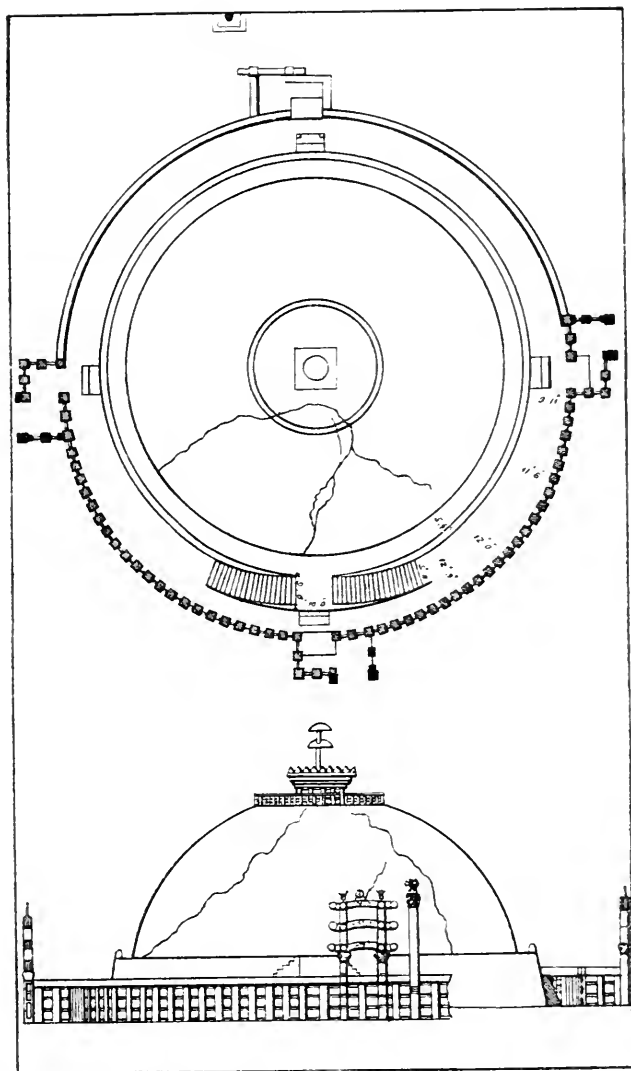
Plan und Seitenansicht des großen Stûpa von Sântschi nach Cunningham, The Bhilsa Topes, Tafel VIII. London 1854.
