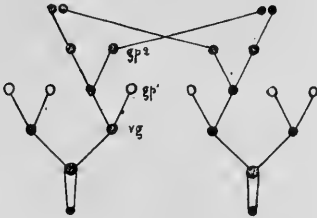
Paramecium caudatum.
