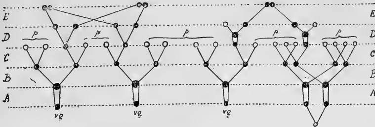
1 er Gamète.
