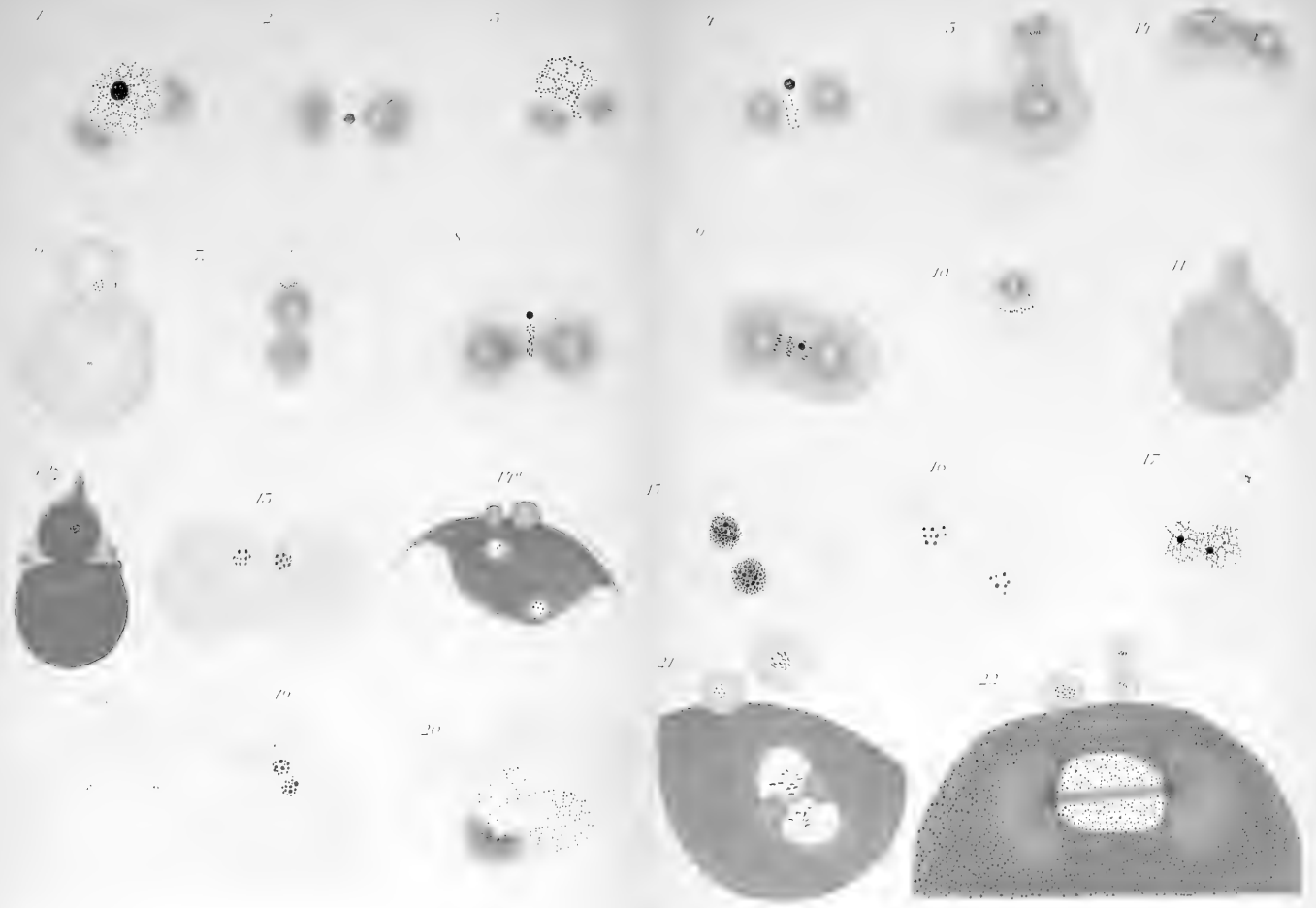
HELIX ASPERSA.
