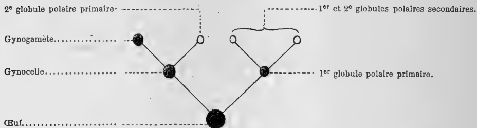
SCHÉMA I.
