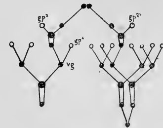
SCHÉMA V.
