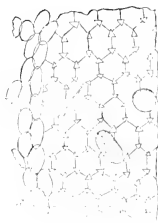
Fig. 2', coupe transversale : di. , portion de diaphragme attachée sur un de ses côtés au parenchyme pariétal des lacunes ; sur le diaphragme, qui présente sa face supérieure, s'élève une moitié de cristal qui, complet, est une double pyramide à 4 faces, une utricule à raphides et une utricule encore vide de tous cristaux.
