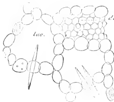
Fig. 1. Pontederia crassipes . — Coupe transversale (gros) d'un fragment du parenchyme lacuneux du pétiole ; lac., lacunes ; di., diaphragmes coupant les lacunes. Une utricule des parois d'une lacune est traversée par un cristal ; une autre utricule a deux cristaux.
