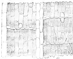
Fig. 2 e et 2'. Pontederia cordata . — 2, coupe longitudinale d'un fragment du parenchyme lacuneux ; di. , diaphragmes traversés par des cristaux perforants et portant des cellules oviformes à raphides, etc.
