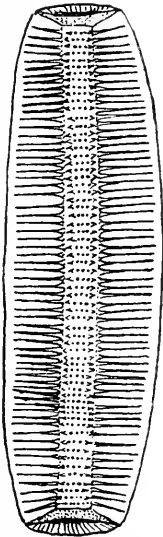
FIG. 23.—Ductus ejaculatorius.
