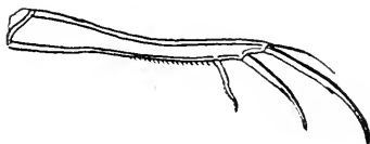
FIG. 6.—Furca.
