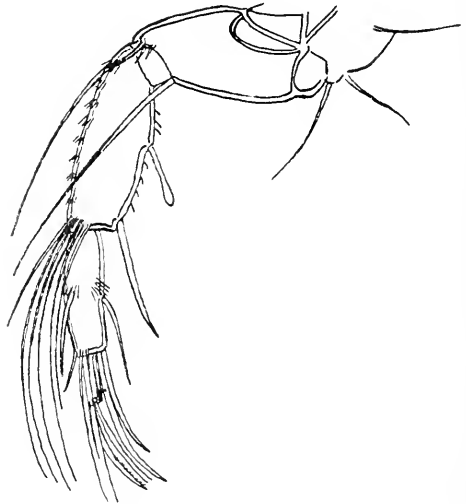
FIG. 3.— Second antenna.
